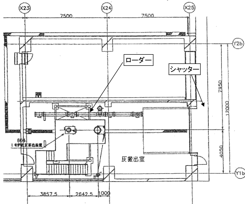
平面図
