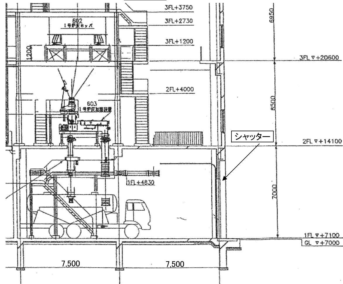
立面図
