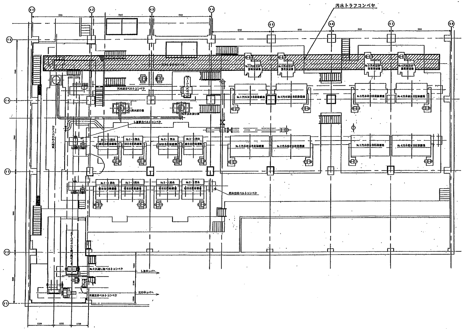
第1処理施設沈砂池平面図
