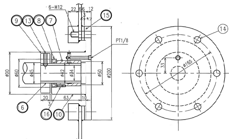
軸受部詳細
