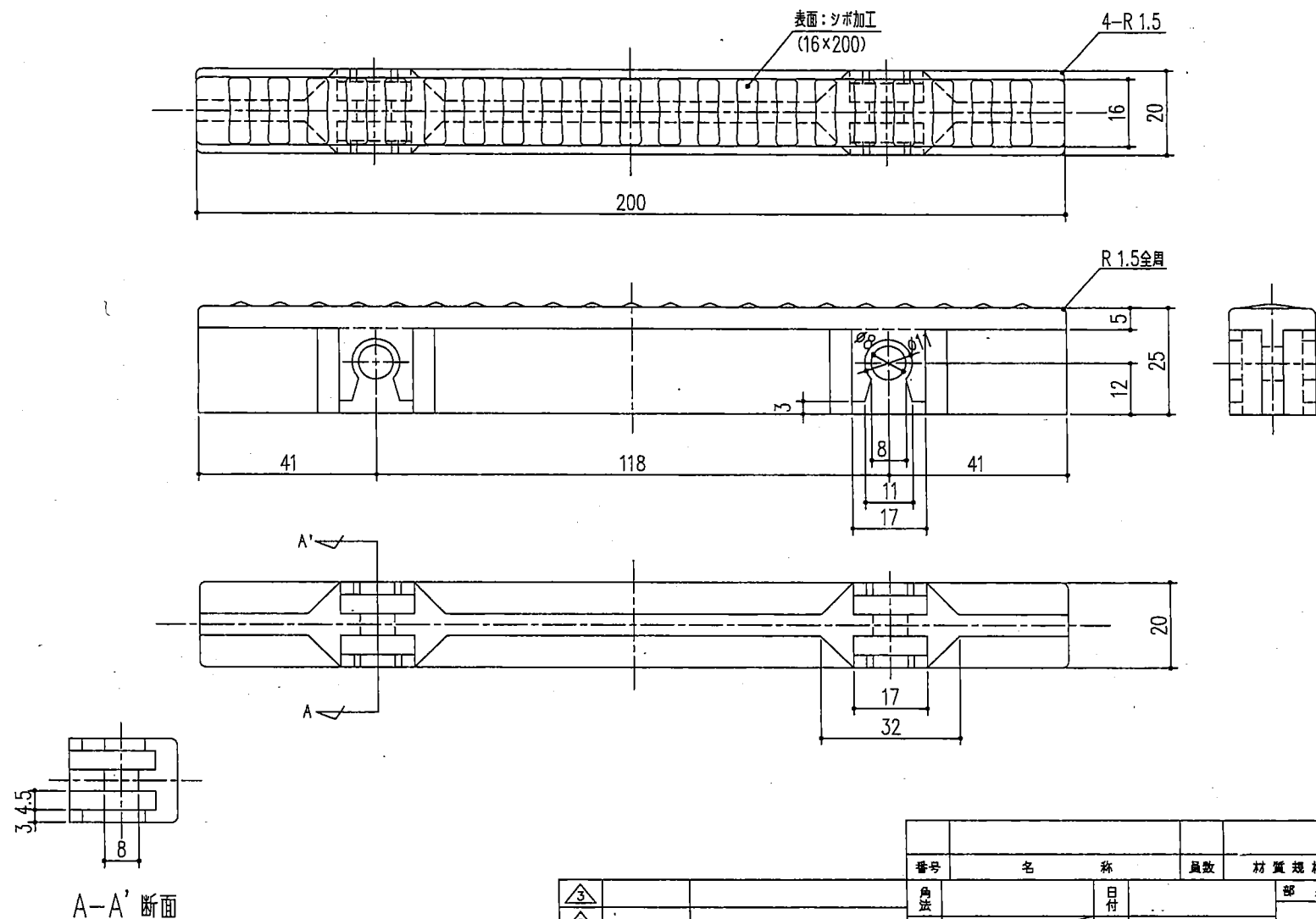
本体詳細図
