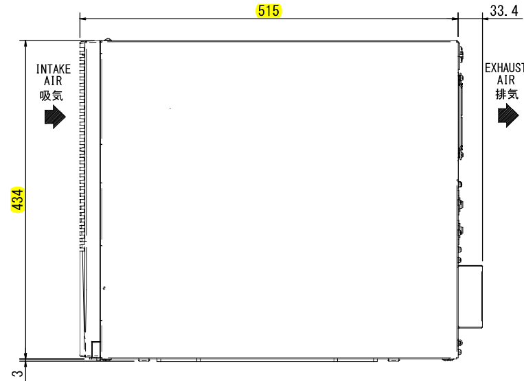
RIGHT SIDE VIEW 右側面
