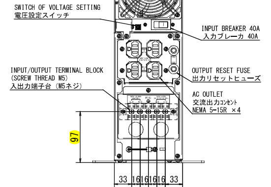
REAR VIEW 背面
