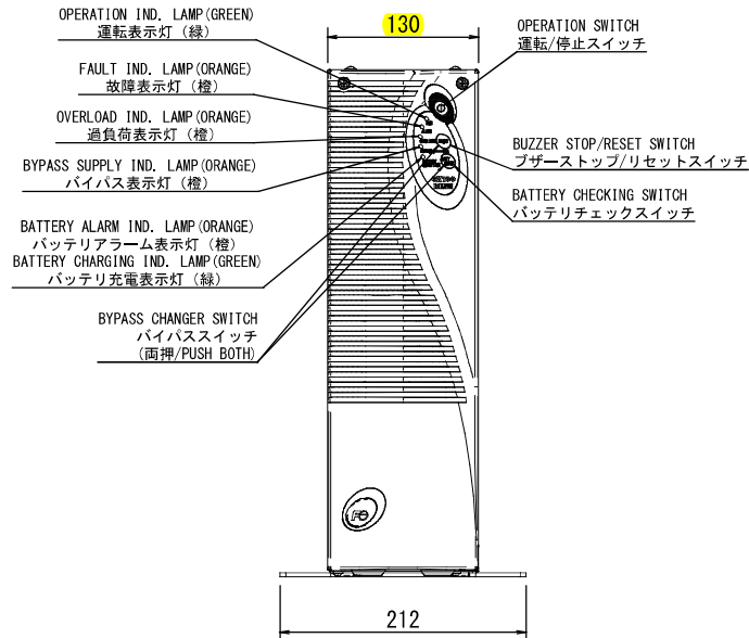
FRONT VIEW 正面
