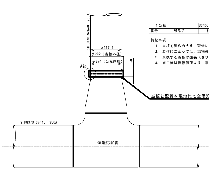
1 系返送汚泥配管修繕図
