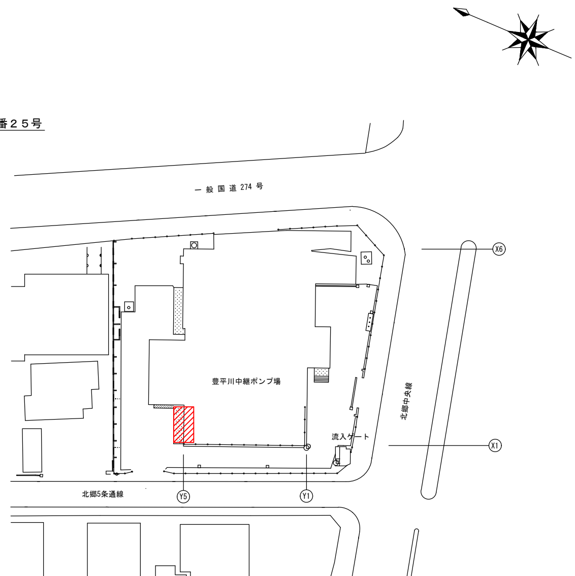
配置図
