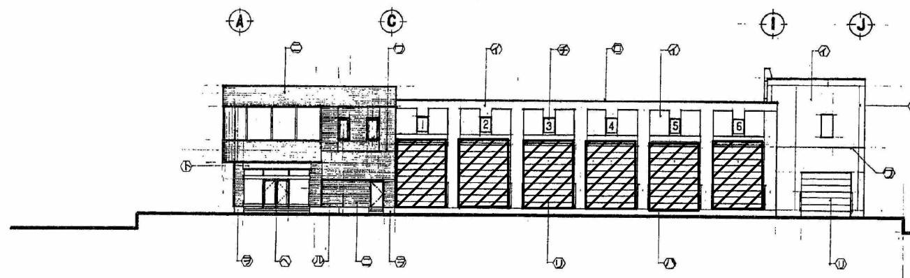
南立面図 (S=Free)
