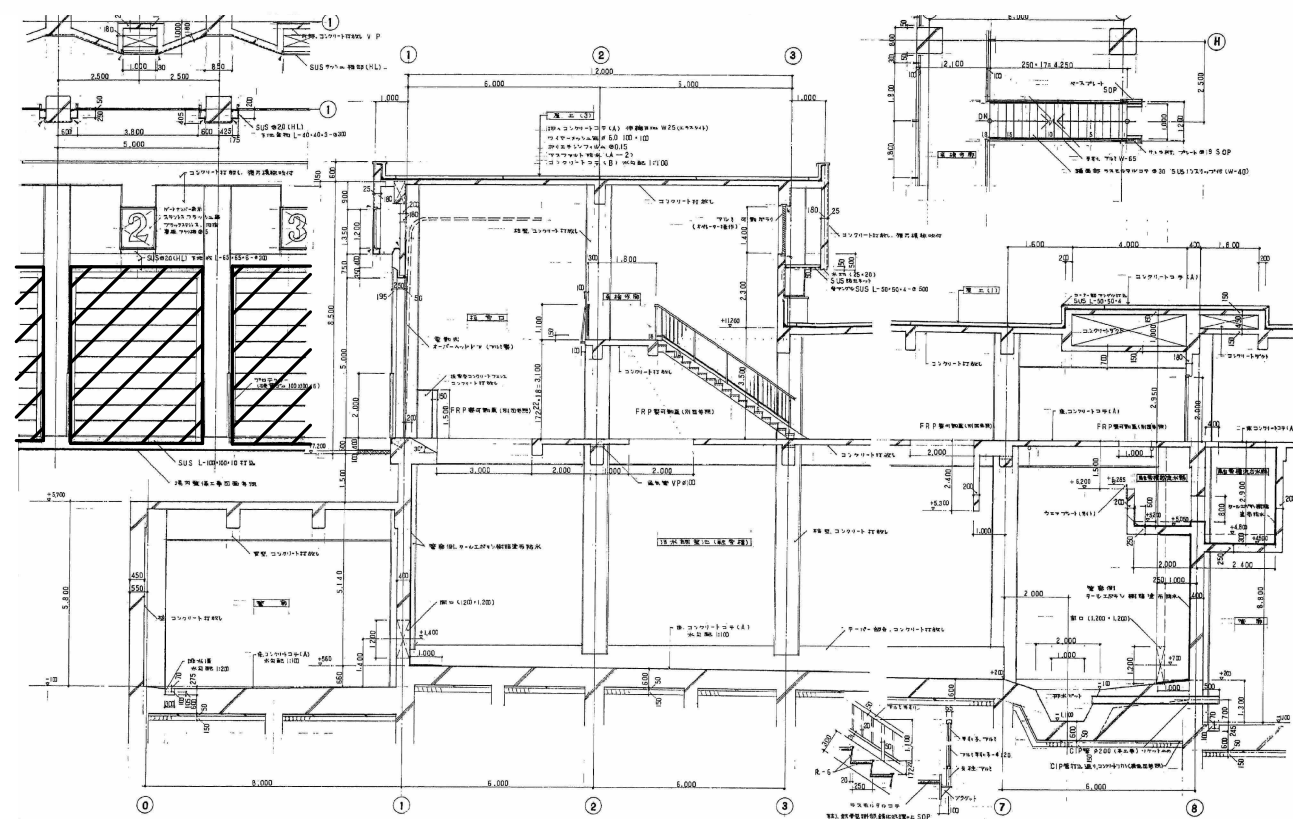
矩形図 (S=Free)
