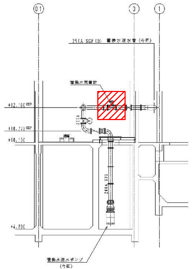
A-A 断面図
