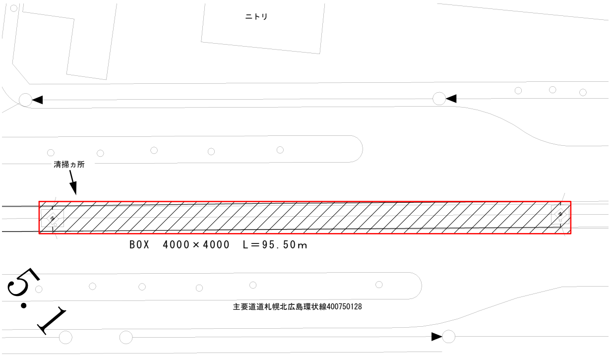
平面図 1 : 500
