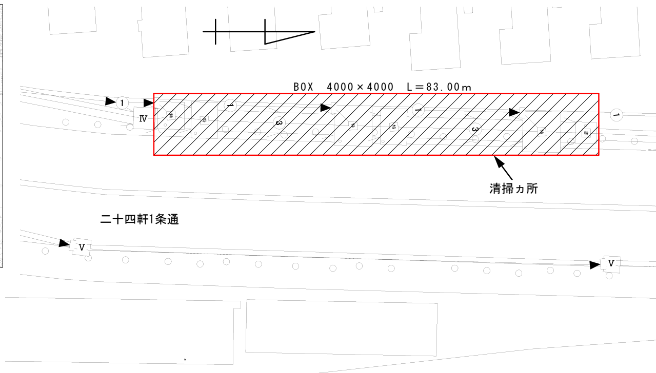
平面図 1 : 500
