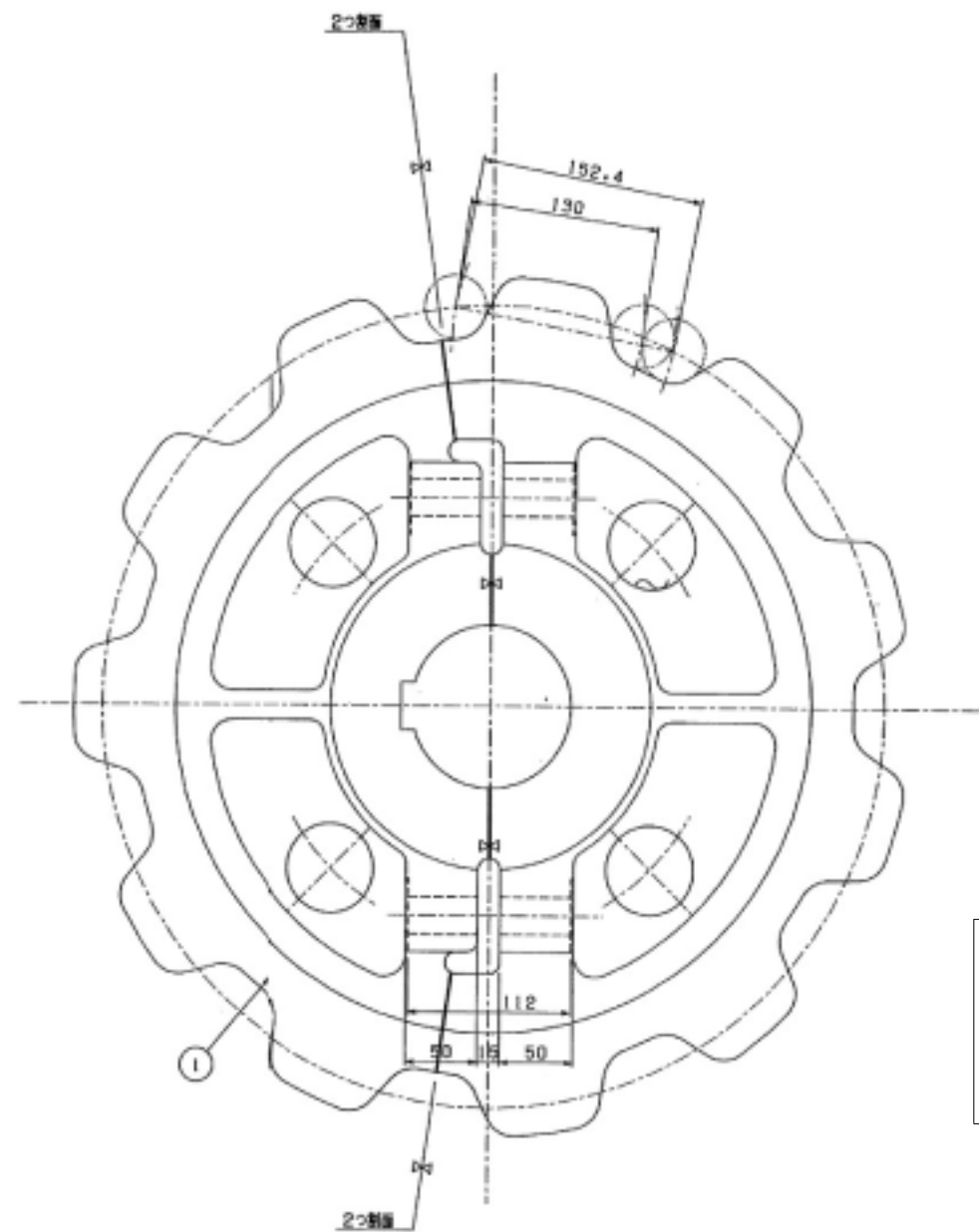
掻揚スプロケット
