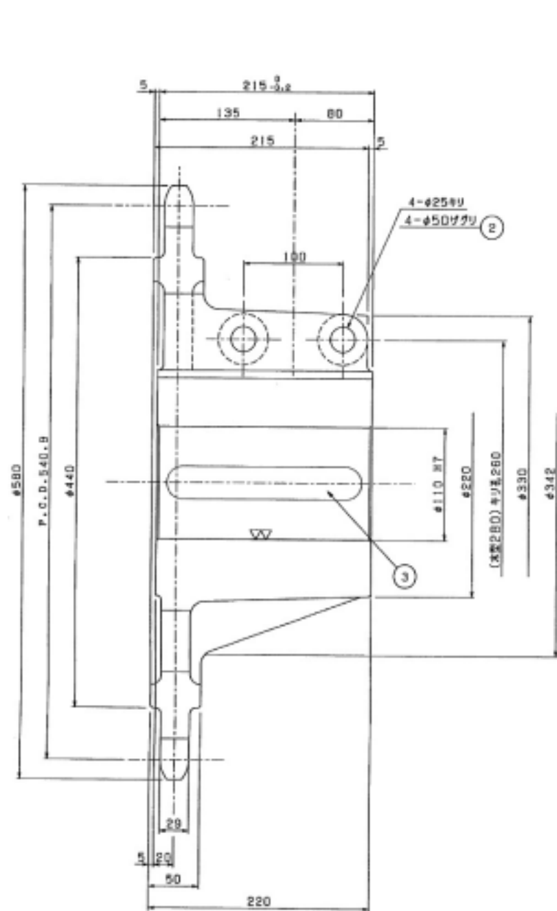
掻揚スプロケット
