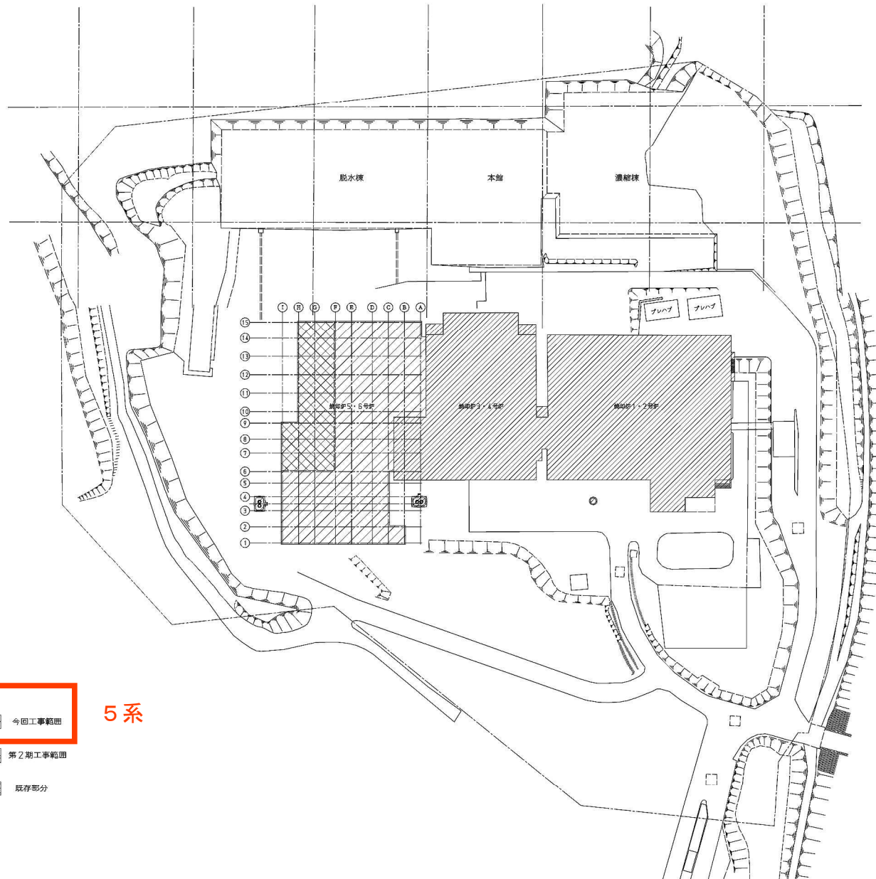
全体配置図 S=1/800
