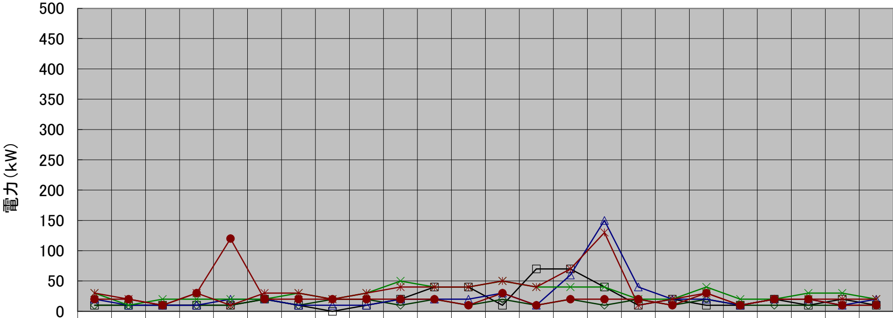
厚別水再生プラザ汚水調整池 月別最大負荷日ロードカーブ(令和6年度上期)
