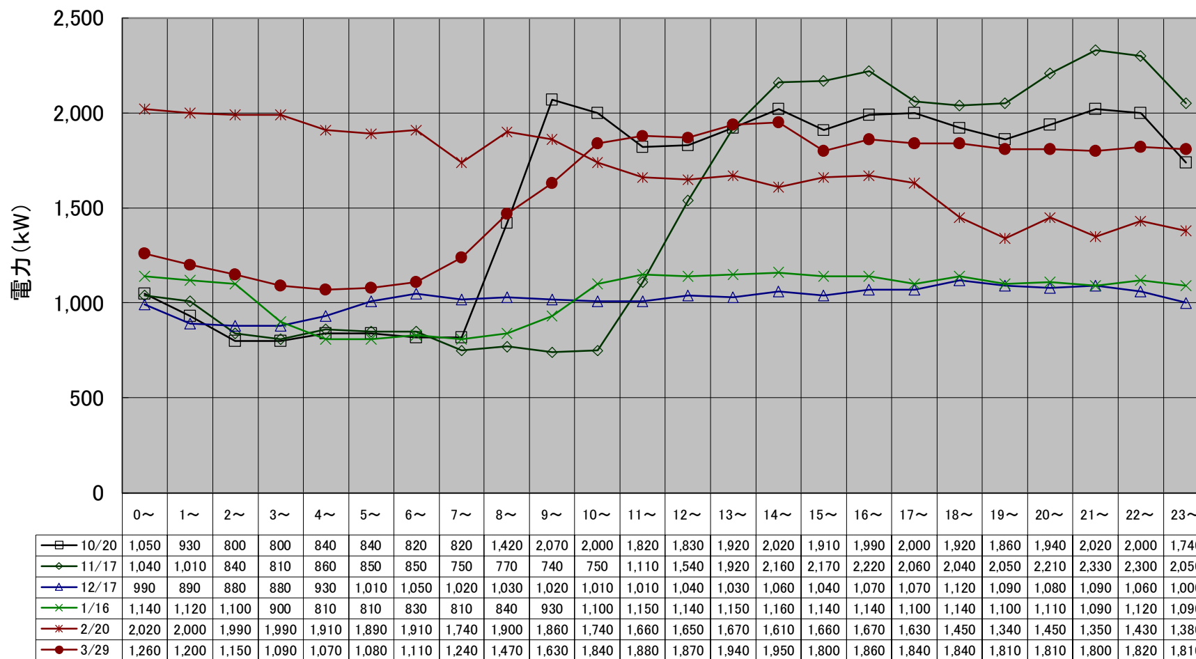
茨戸水再生プラザ 月別最大負荷日ロードカーブ(令和5年度下期)
