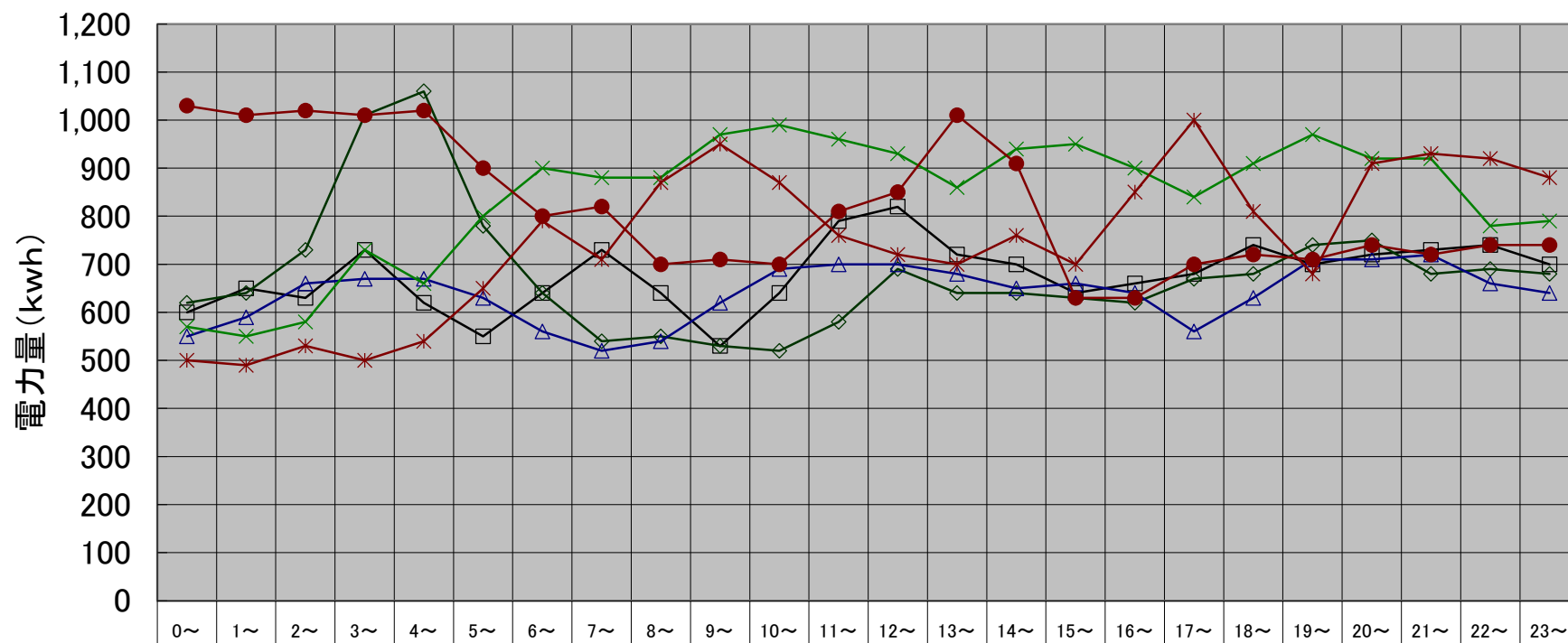
伏古川水再生プラザ 月別最大負荷日ロードカーブ(令和6年度上期)
