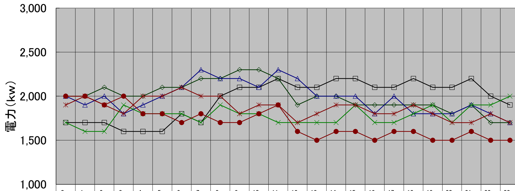
西部スラッジセンター 月別最大負荷日ロードカーブ(令和5年度下期)
