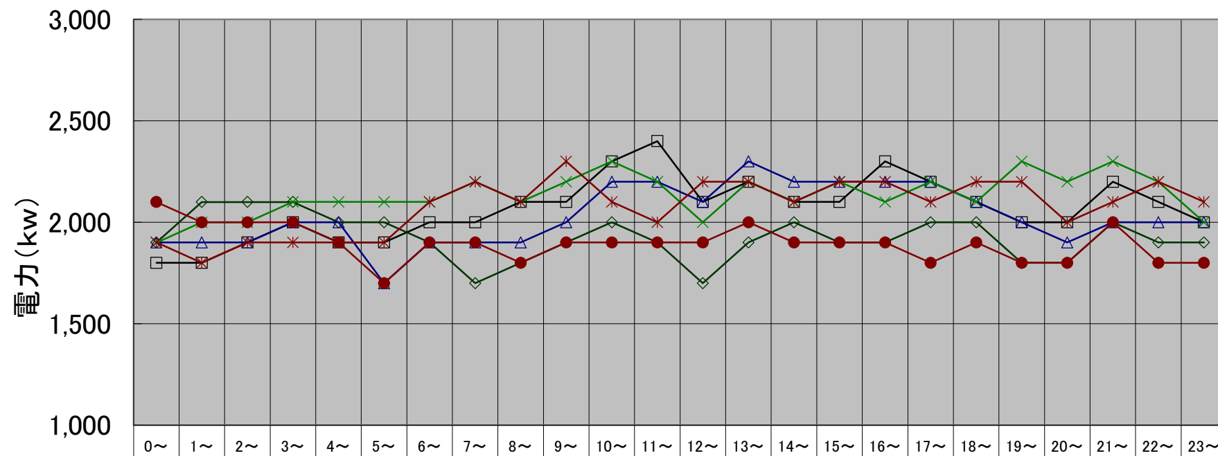
西部スラッジセンター 月別最大負荷日ロードカーブ(令和6年度上期)
