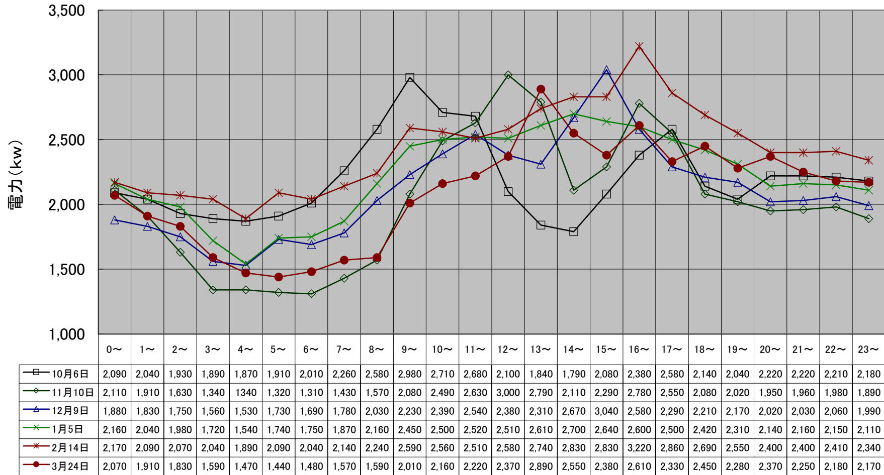
創成川水再生プラザ 月別最大負荷日ロードカーブ(令和5年度下期)
