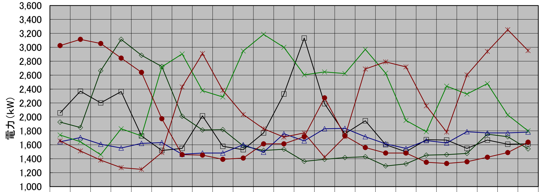
豊平川水再生プラザ 月別最大負荷日ロードカーブ(令和6年度上期)
