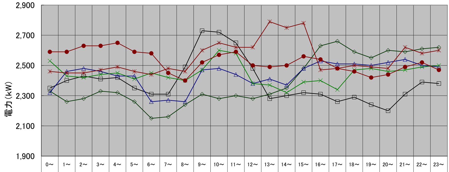
東部水再生プラザ 月別最大負荷日ロードカーブ(令和5年度下期)
