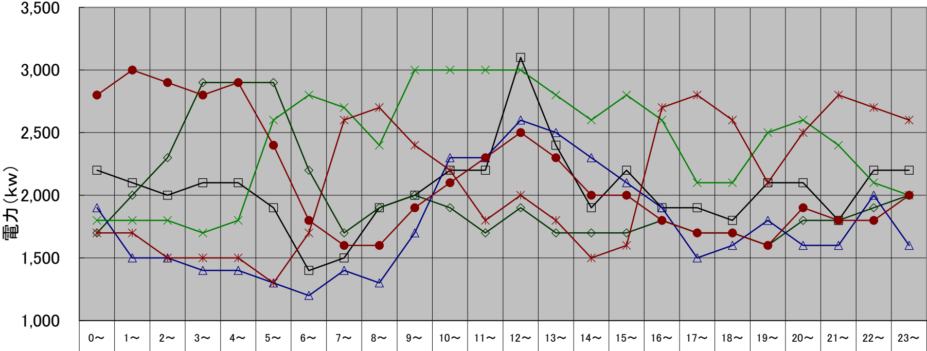
新川水再生プラザ 月別最大負荷日ロードカーブ(令和6年度上期)
