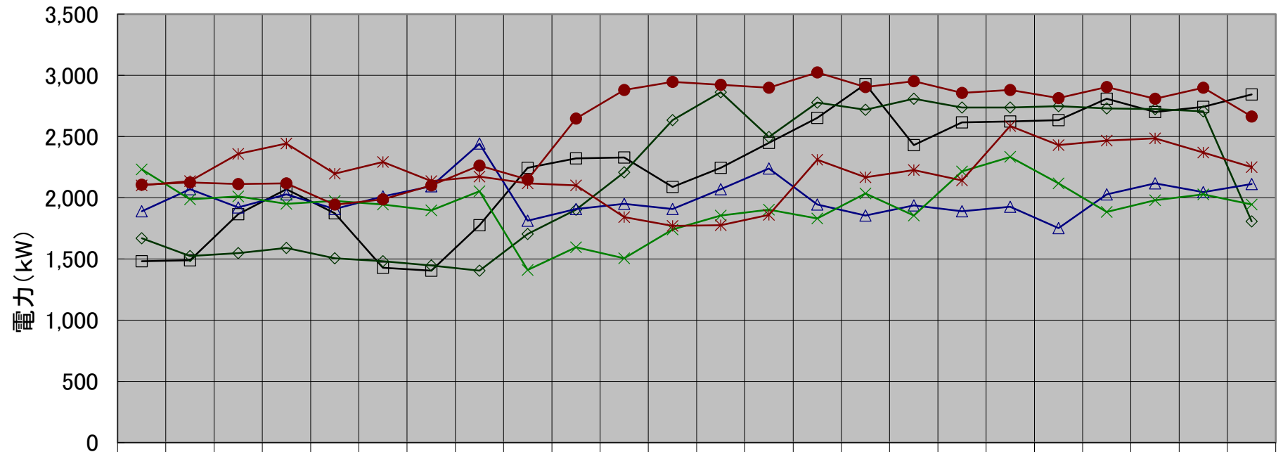
手稲水再生プラザ 月別最大負荷日ロードカーブ(令和5年度下期)
