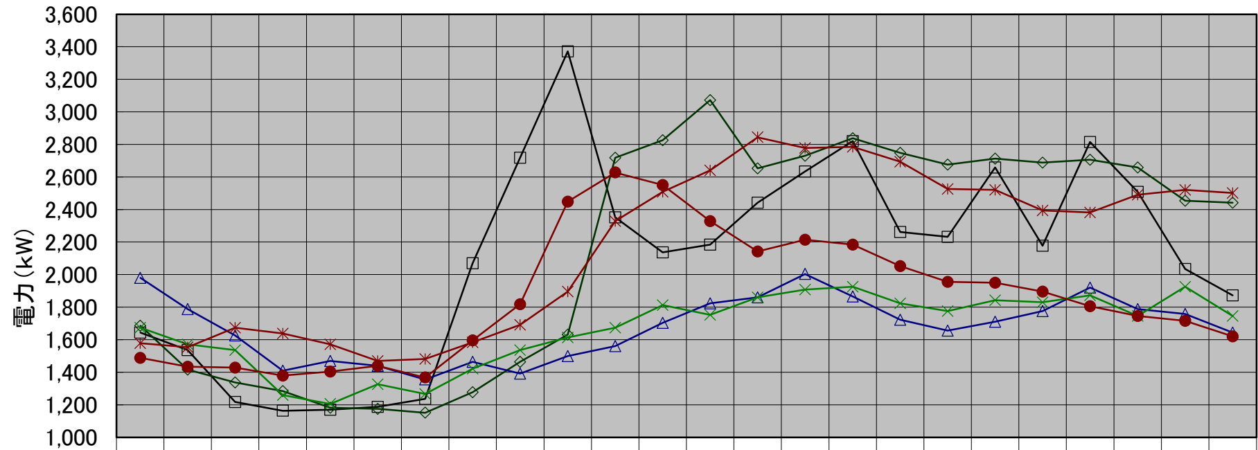
豊平川水再生プラザ 月別最大負荷日ロードカーブ(令和5年度下期)
