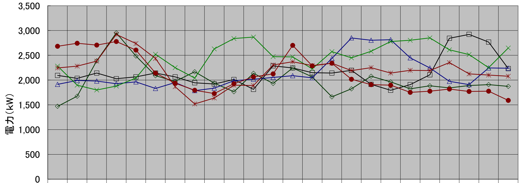
手稲水再生プラザ 月別最大負荷日ロードカーブ(令和6年度上期)
