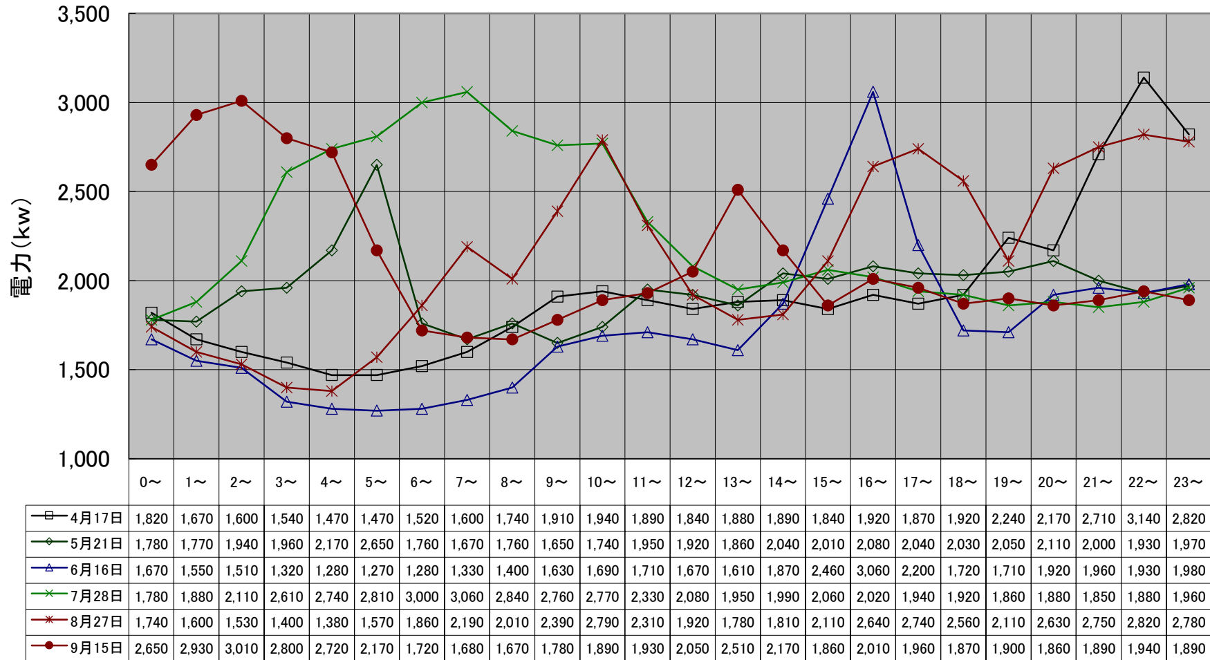
創成川水再生プラザ 月別最大負荷日ロードカーブ(令和6年度上期)
