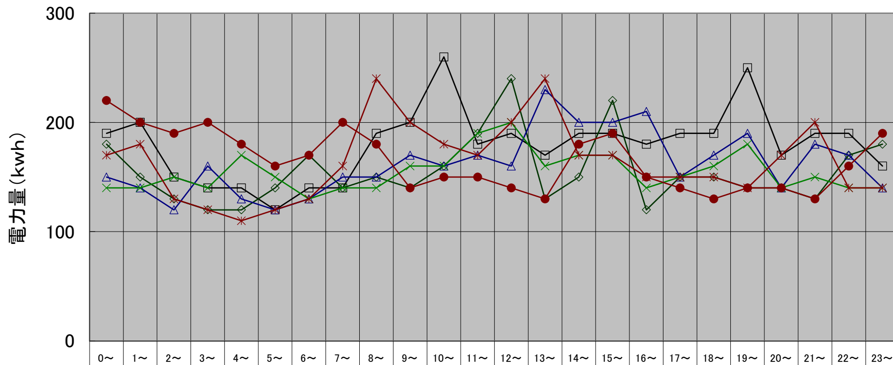
拓北水再生プラザ 月別最大負荷日ロードカーブ(令和6年度上期)
