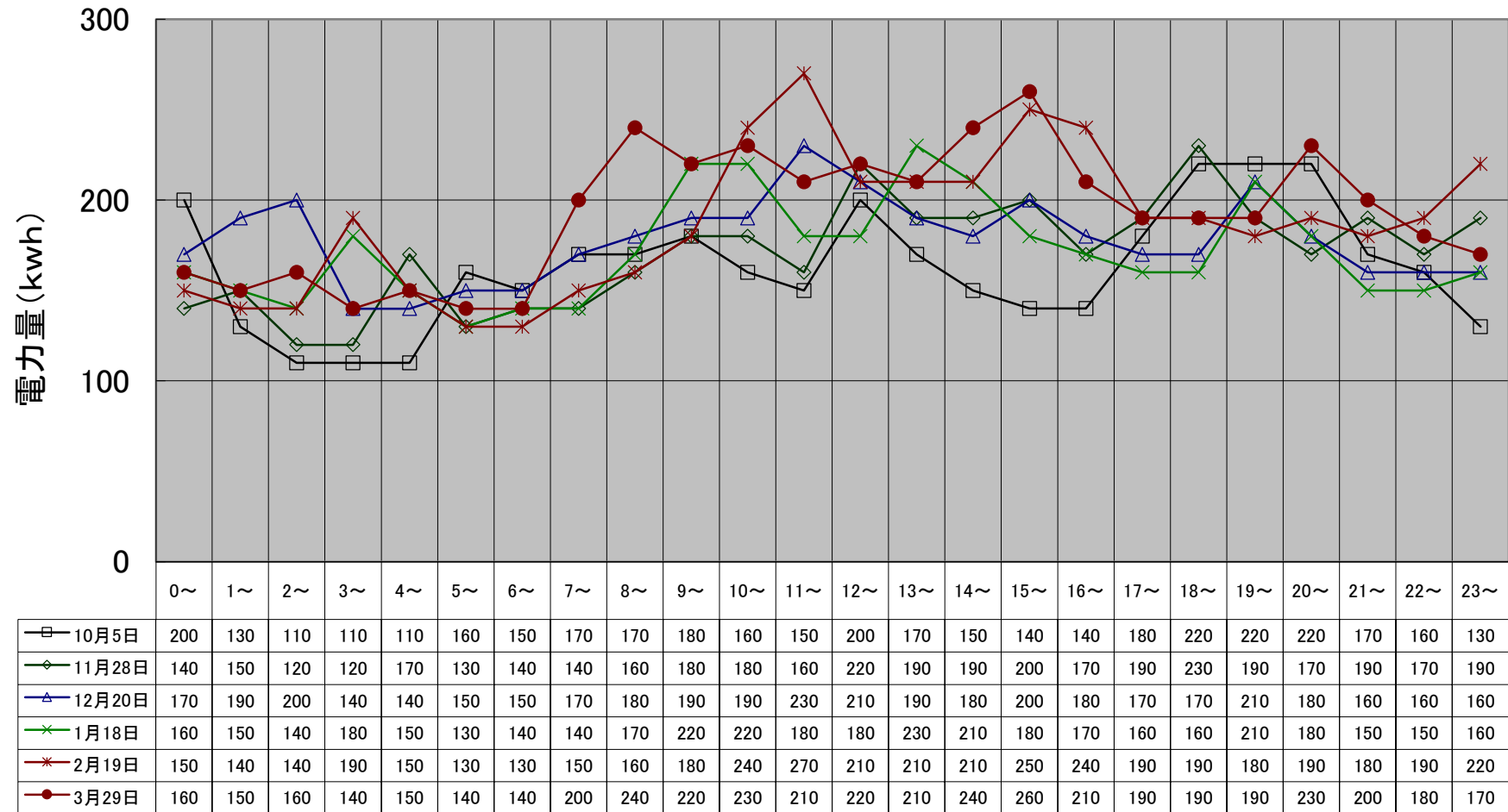
拓北水再生プラザ 月別最大負荷日ロードカーブ(令和5年度下期)
