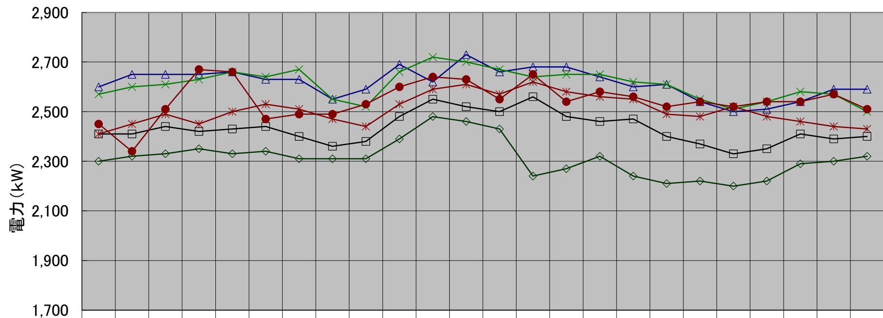
東部水再生プラザ 月別最大負荷日ロードカーブ(令和6年度上期)
