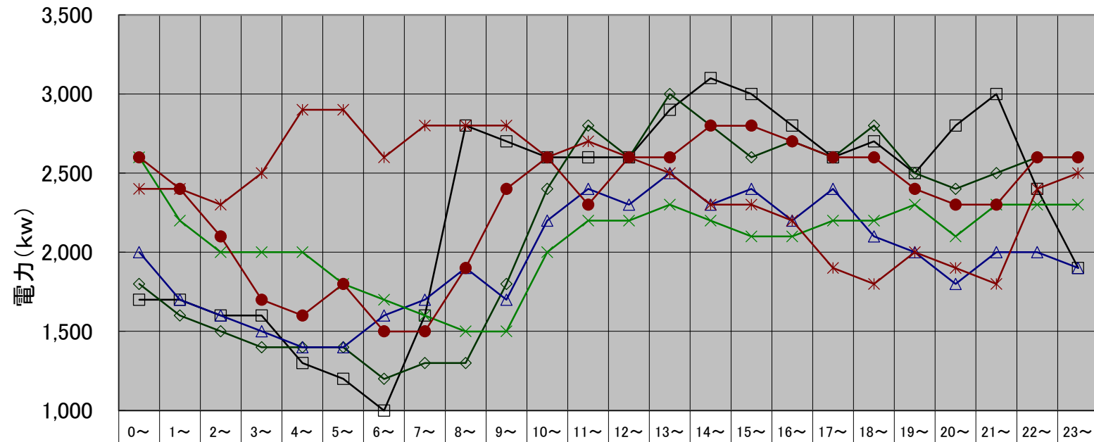
新川水再生プラザ 月別最大負荷日ロードカーブ(令和5年度下期)
