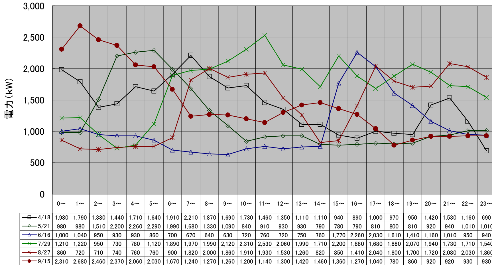
茨戸水再生プラザ 月別最大負荷日ロードカーブ(令和6年度上期)
