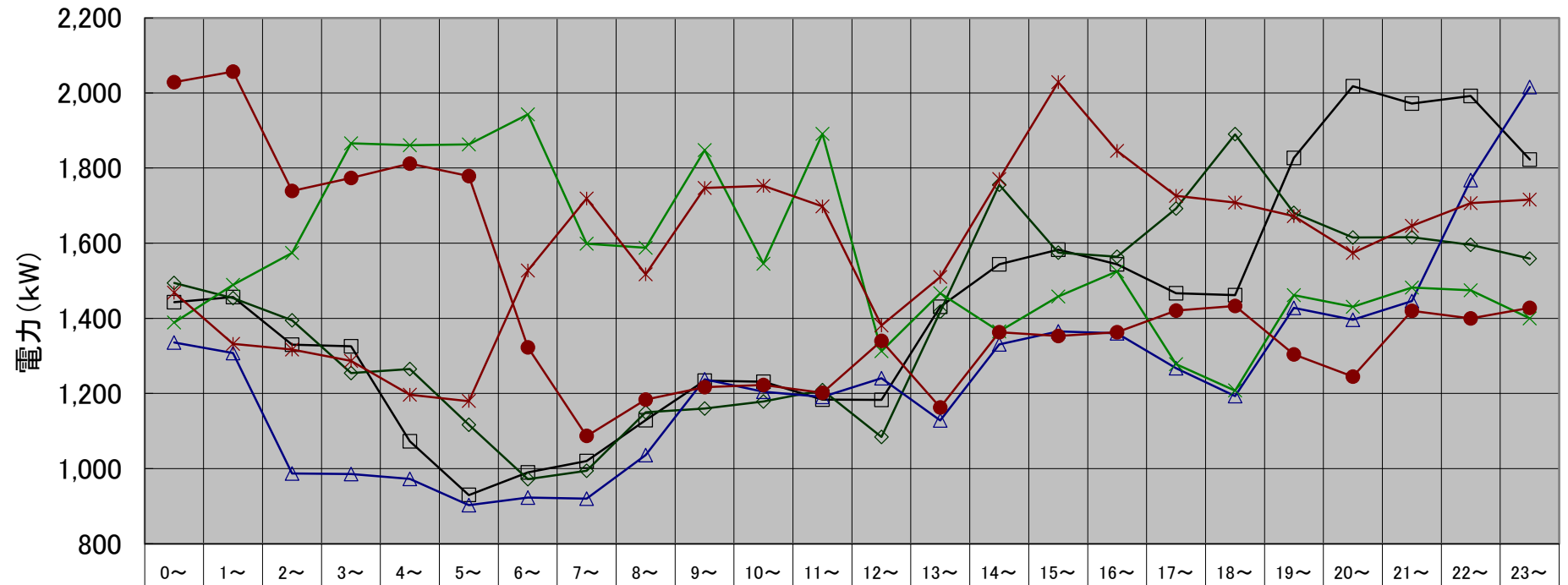
厚別水再生プラザ 月別最大負荷日ロードカーブ(令和6年度上期)
