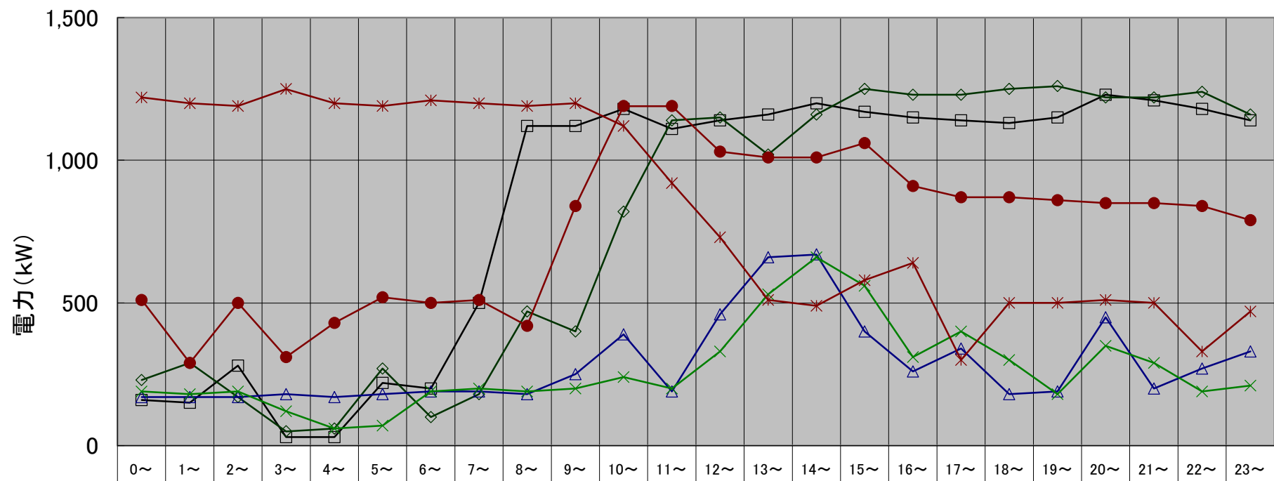
手稲中継ポンプ場 月別最大負荷日ロードカーブ(令和5年度下期)
