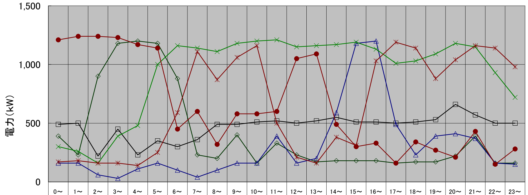
手稲中継ポンプ場 月別最大負荷日ロードカーブ(令和6年度上期)
