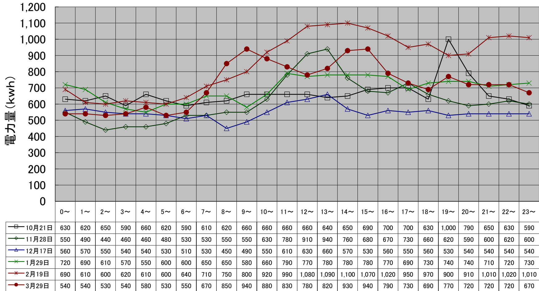
伏古川水再生プラザ 月別最大負荷日ロードカーブ(令和5年度下期)
