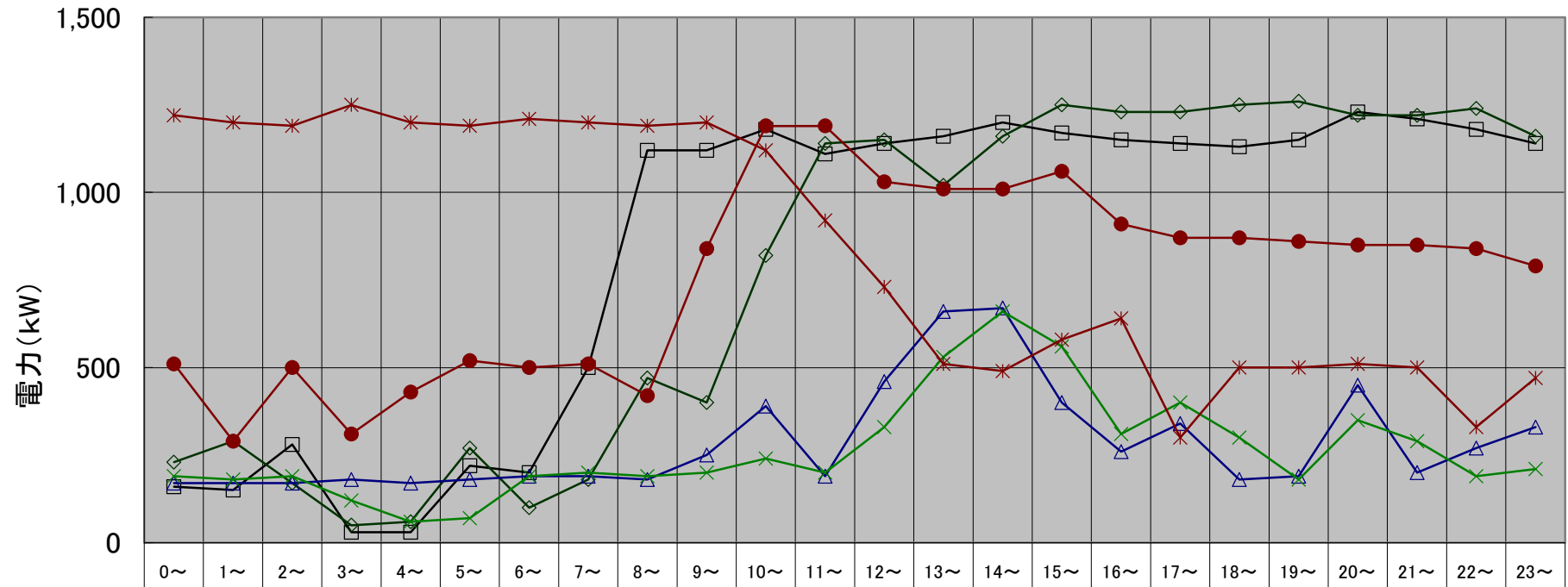
手稲中継ポンプ場 月別最大負荷日ロードカーブ(令和5年度下期)
