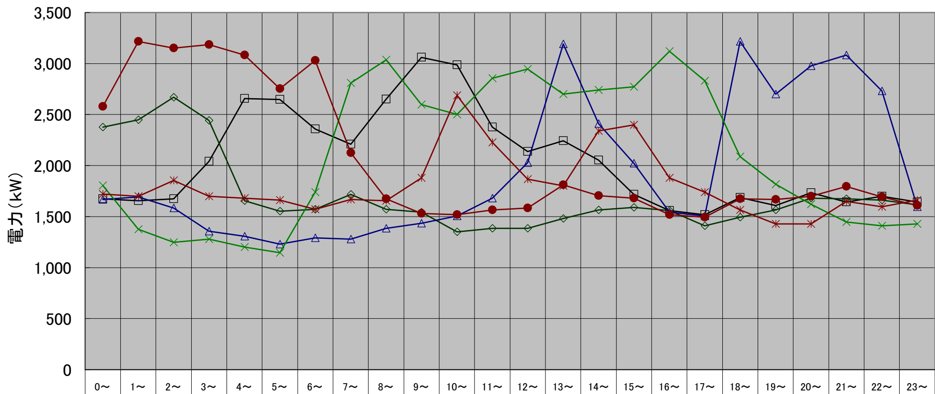
月別最大負荷日ロードカーブ(令和5年度上期)
