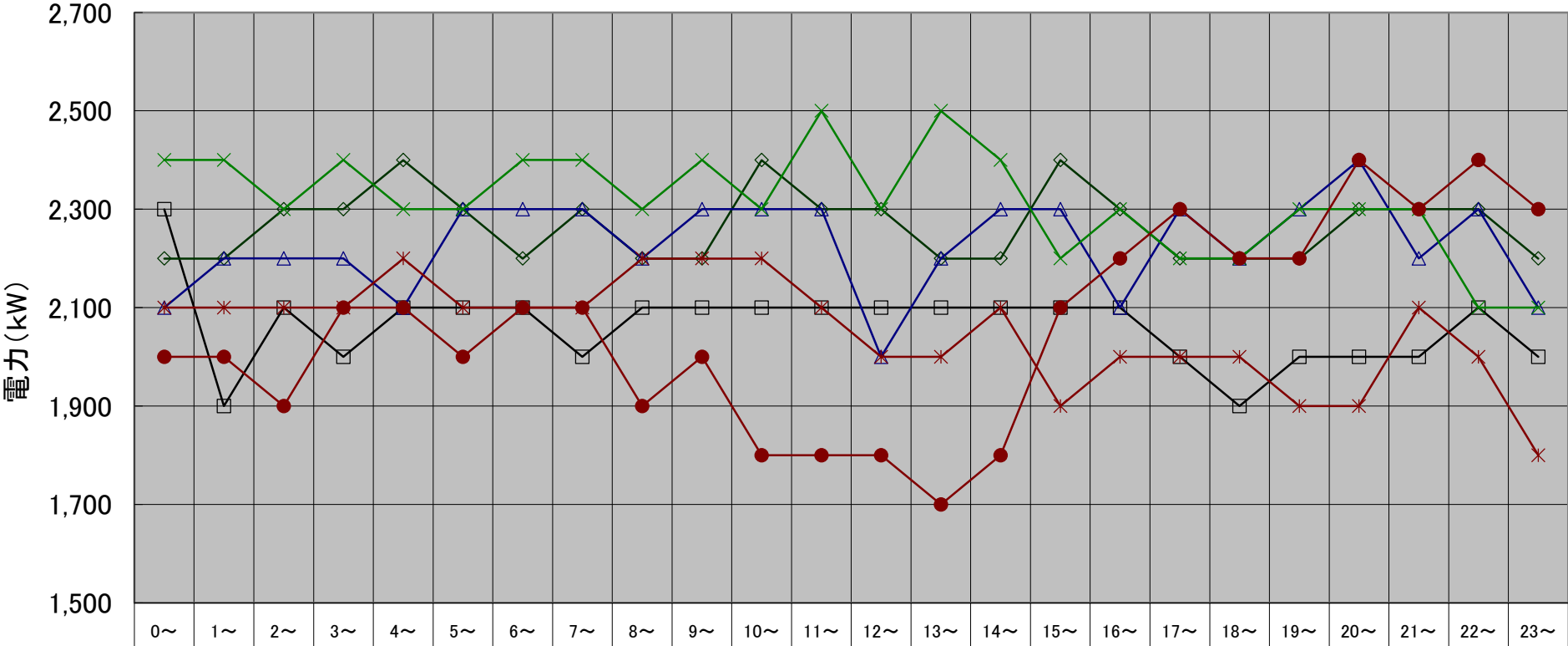
月別最大負荷日ロードカーブ(令和5年度上期)
