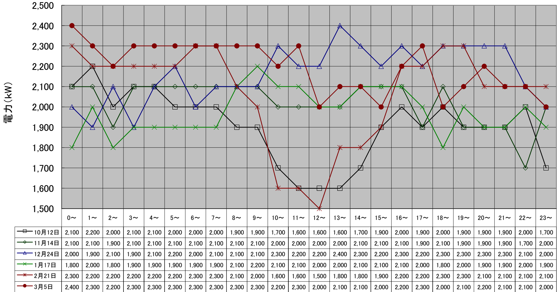
月別最大負荷日ロードカーブ(令和4年度下期)
