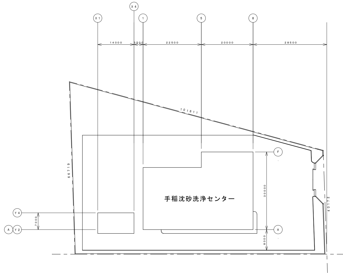
全体配置図
