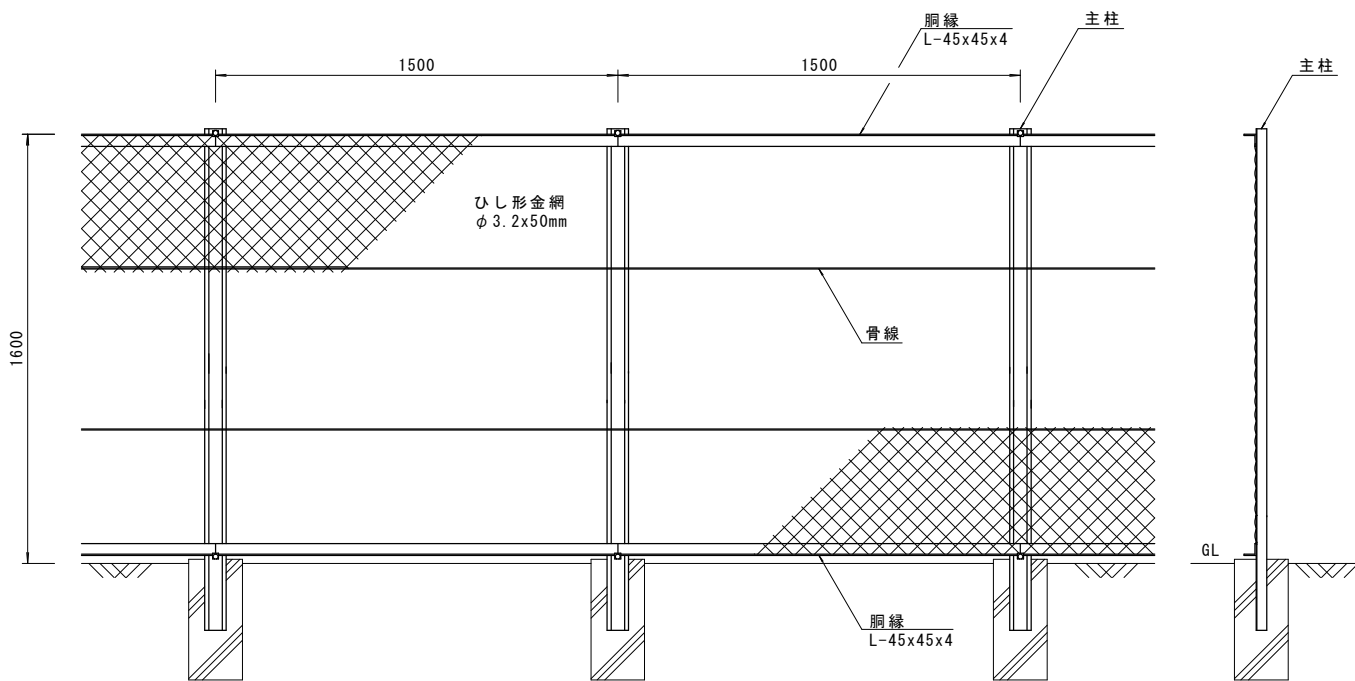
正面図 S=1/20
