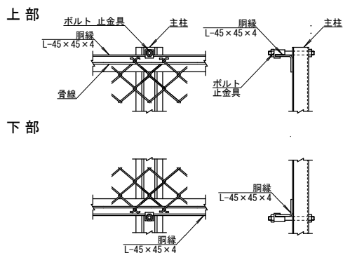
詳細図 S=1/10
