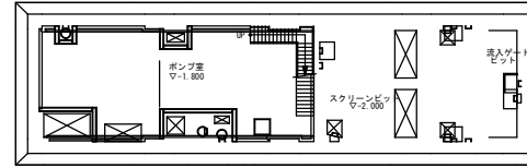
地下1階平面図
