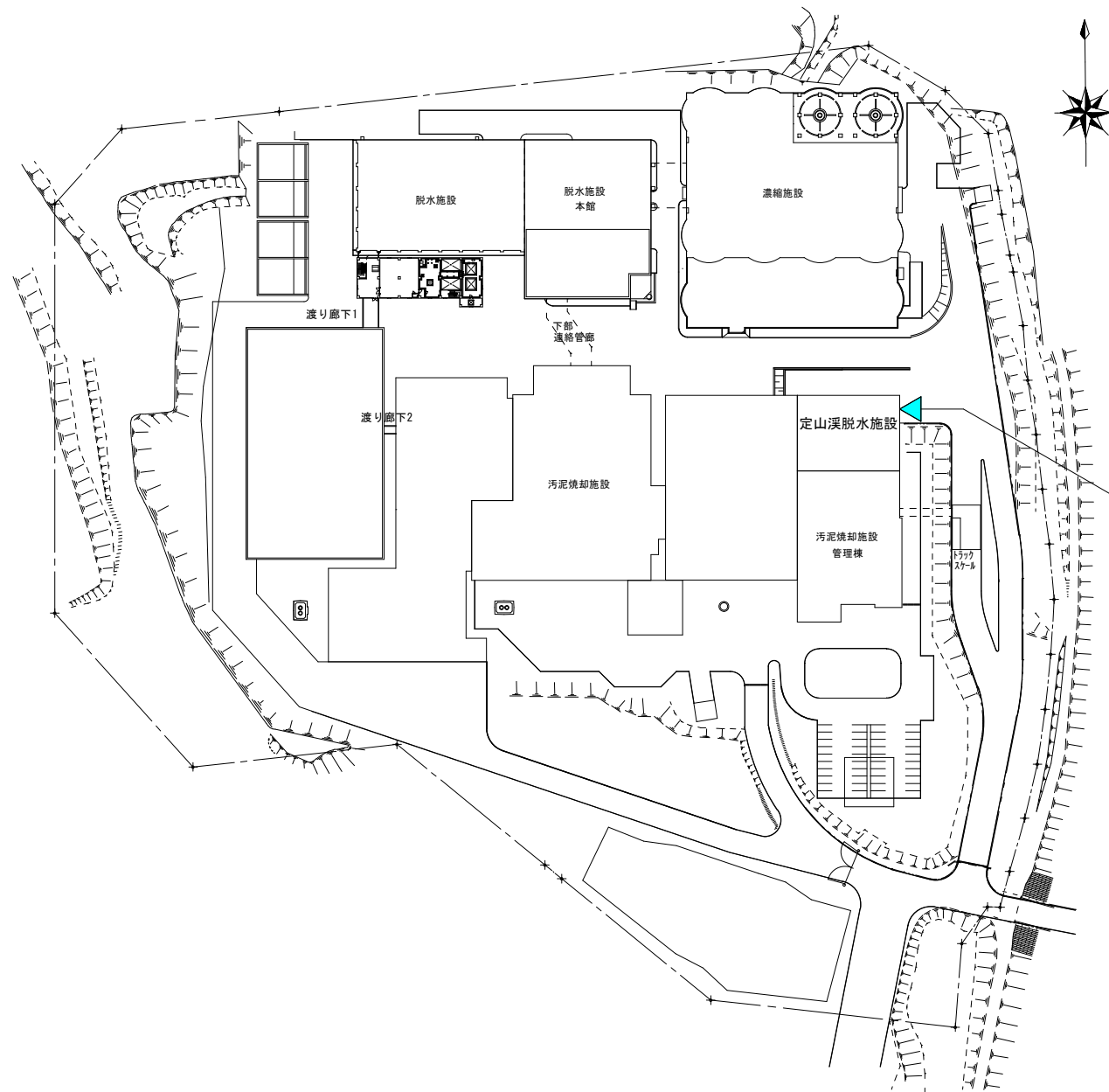
西部スラッジセンター施設平面図
