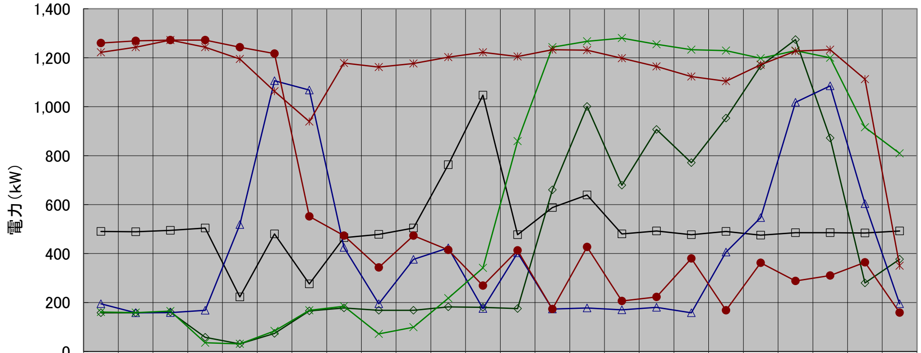
月別最大負荷日ロードカーブ(令和4年度上期)
