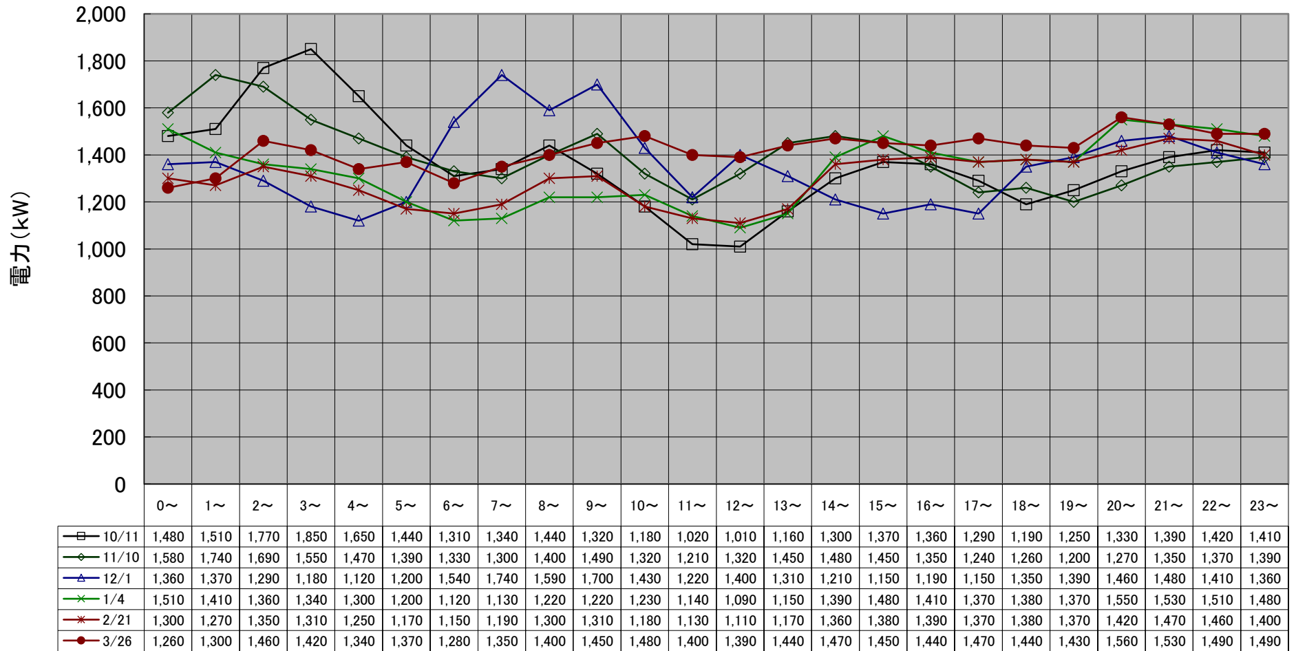
月別最大負荷日ロードカーブ(令和3年度下期)
