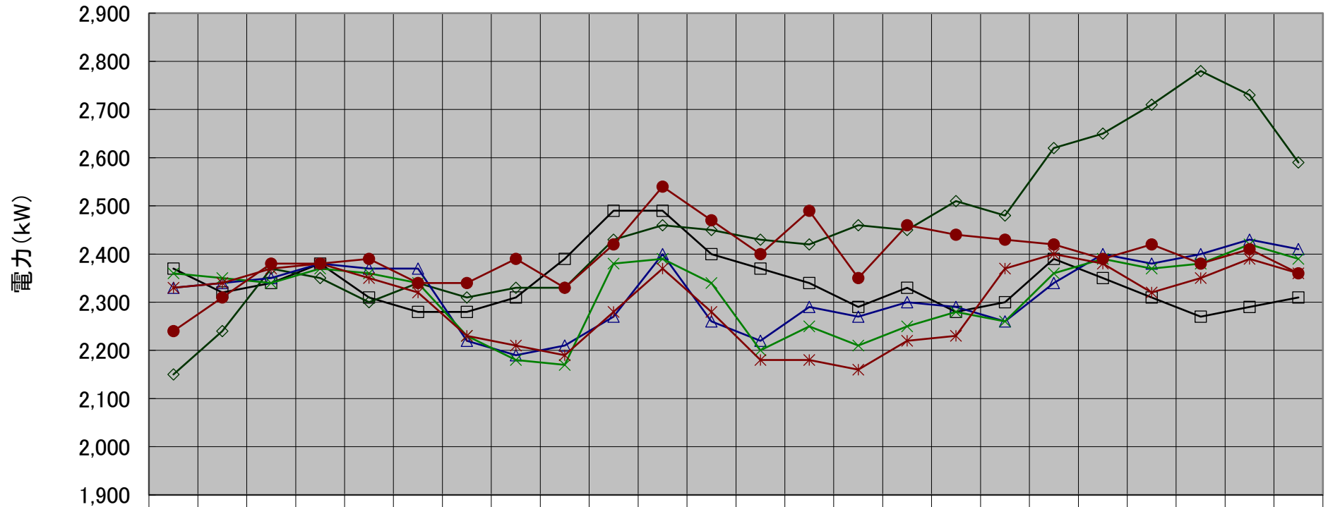
月別最大負荷日ロードカーブ(令和3年度下期)
