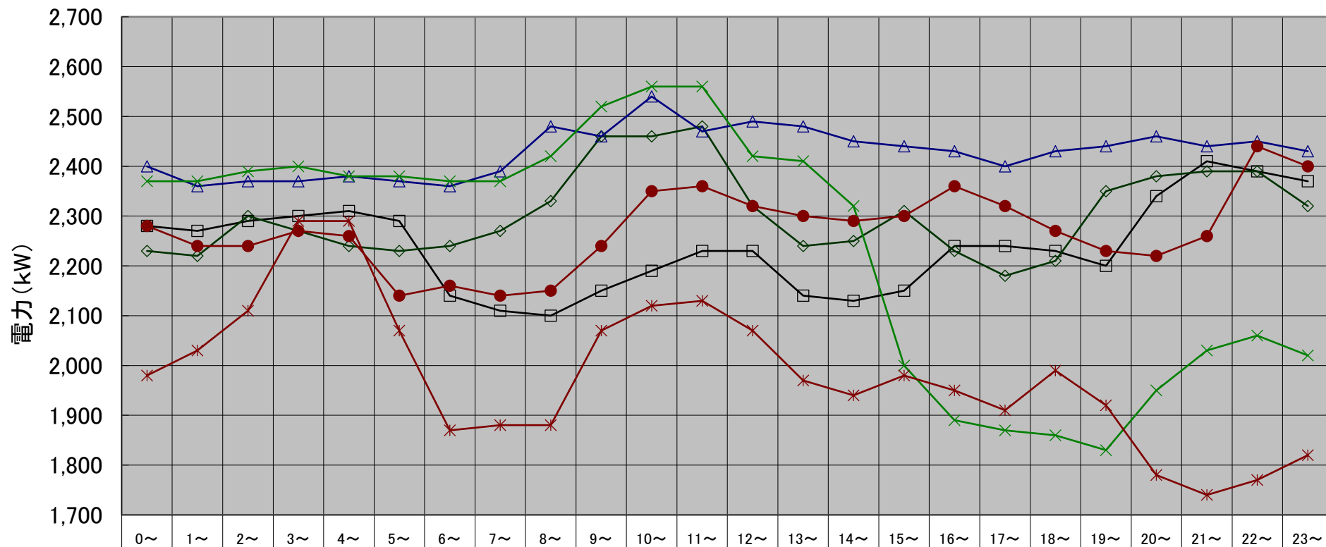
月別最大負荷日ロードカーブ(令和4年度上期)
