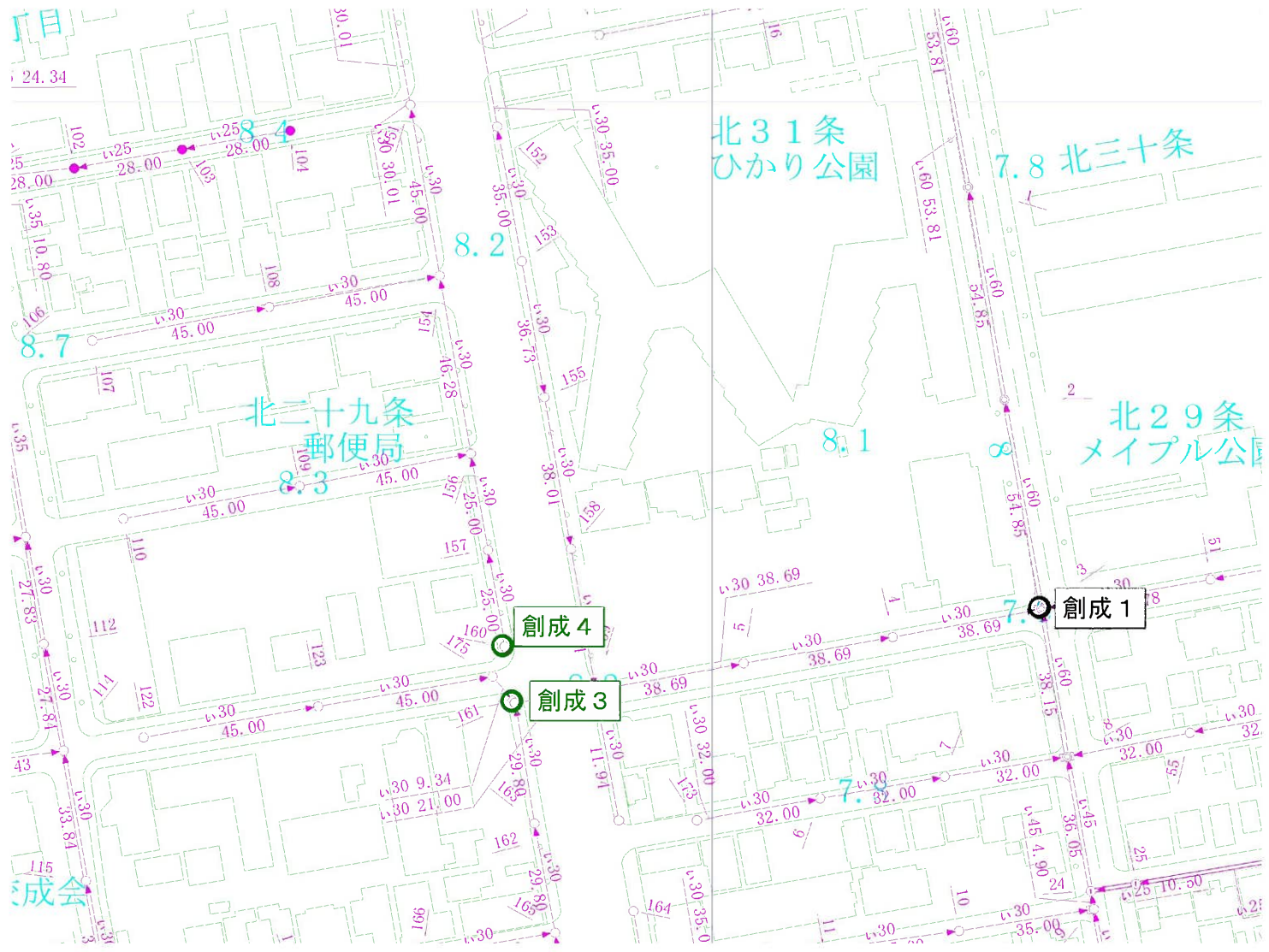
【管路網図】
