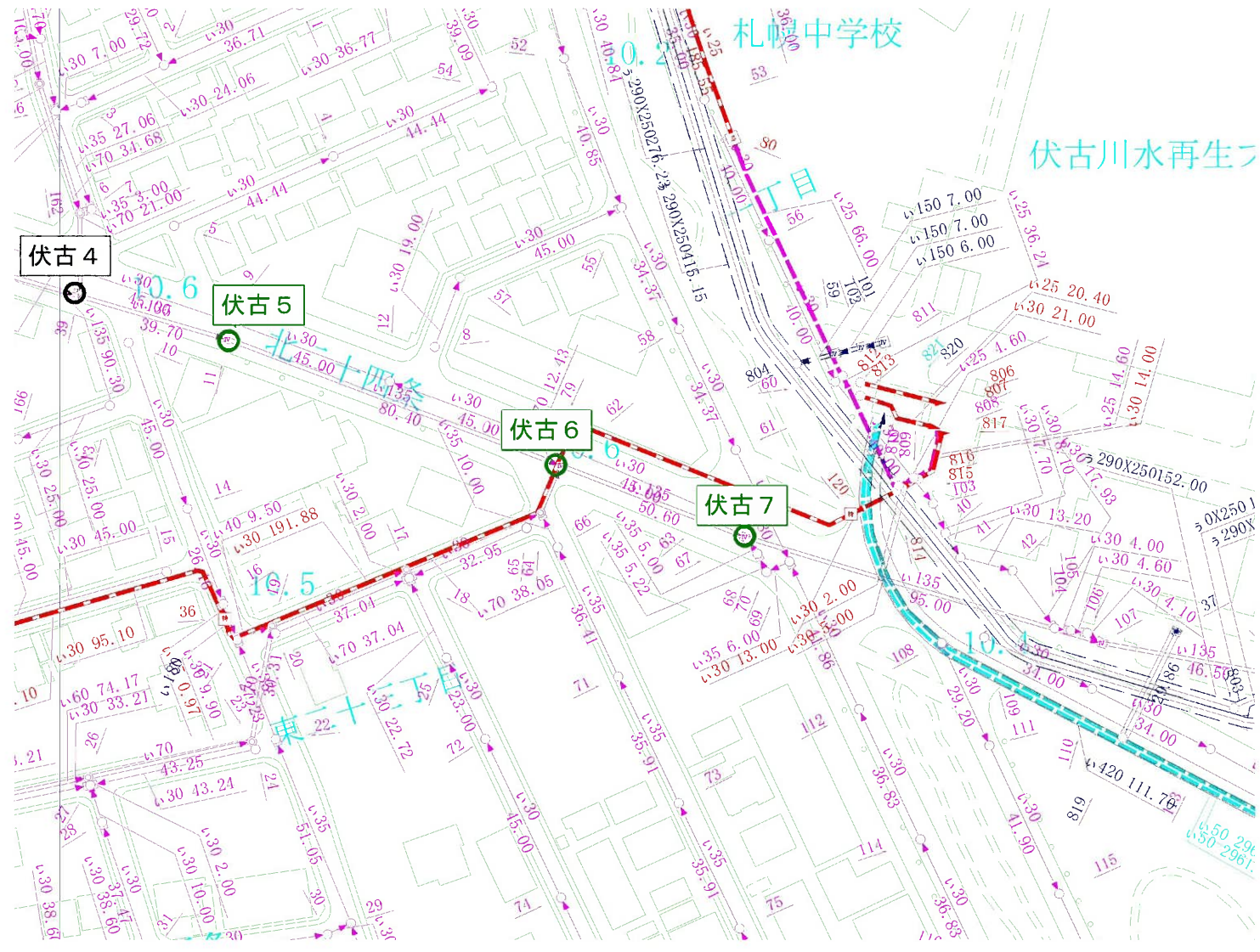
【管路網図】
