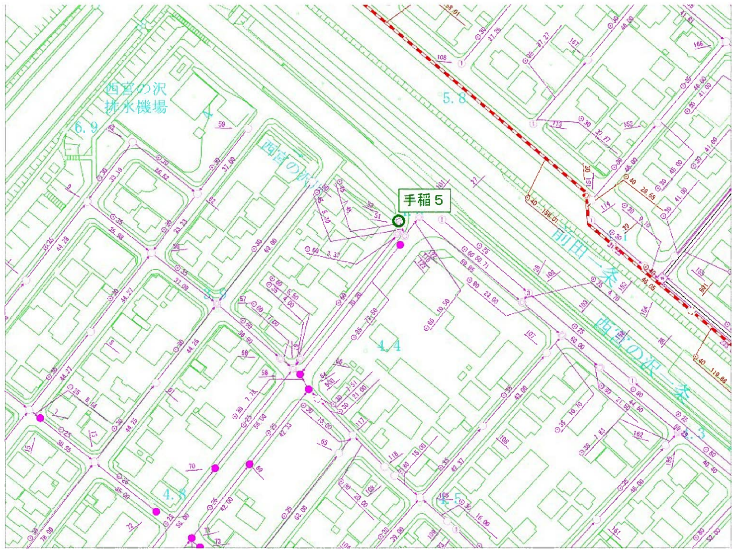
【管路網図】
