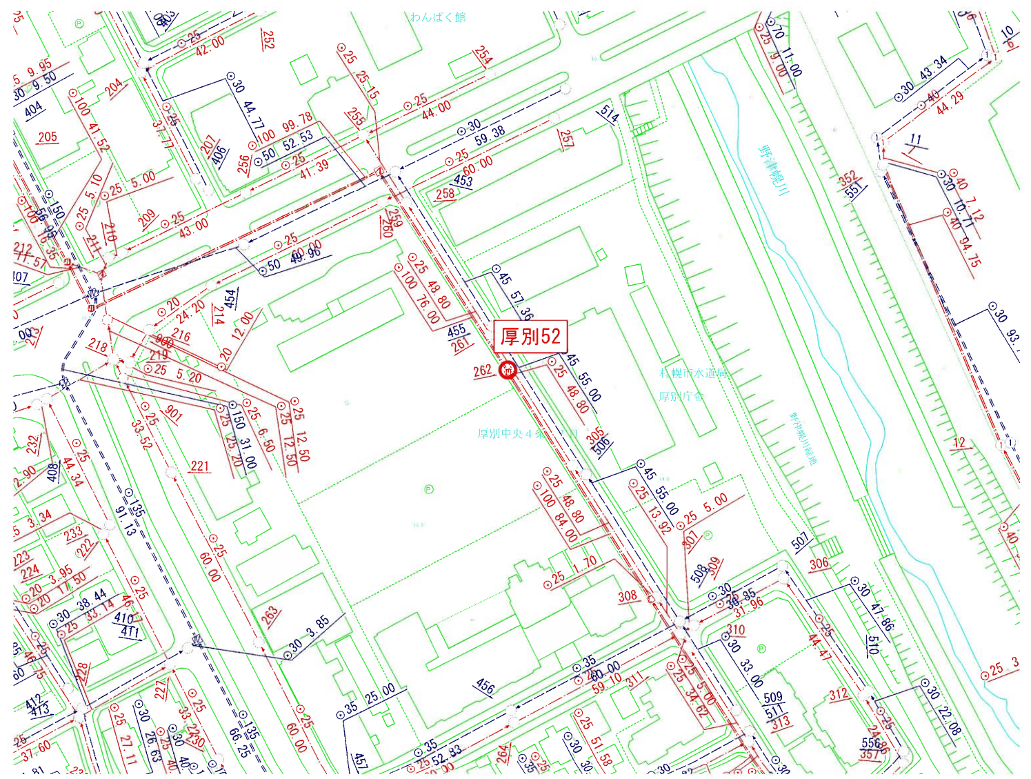
【管路網図】
