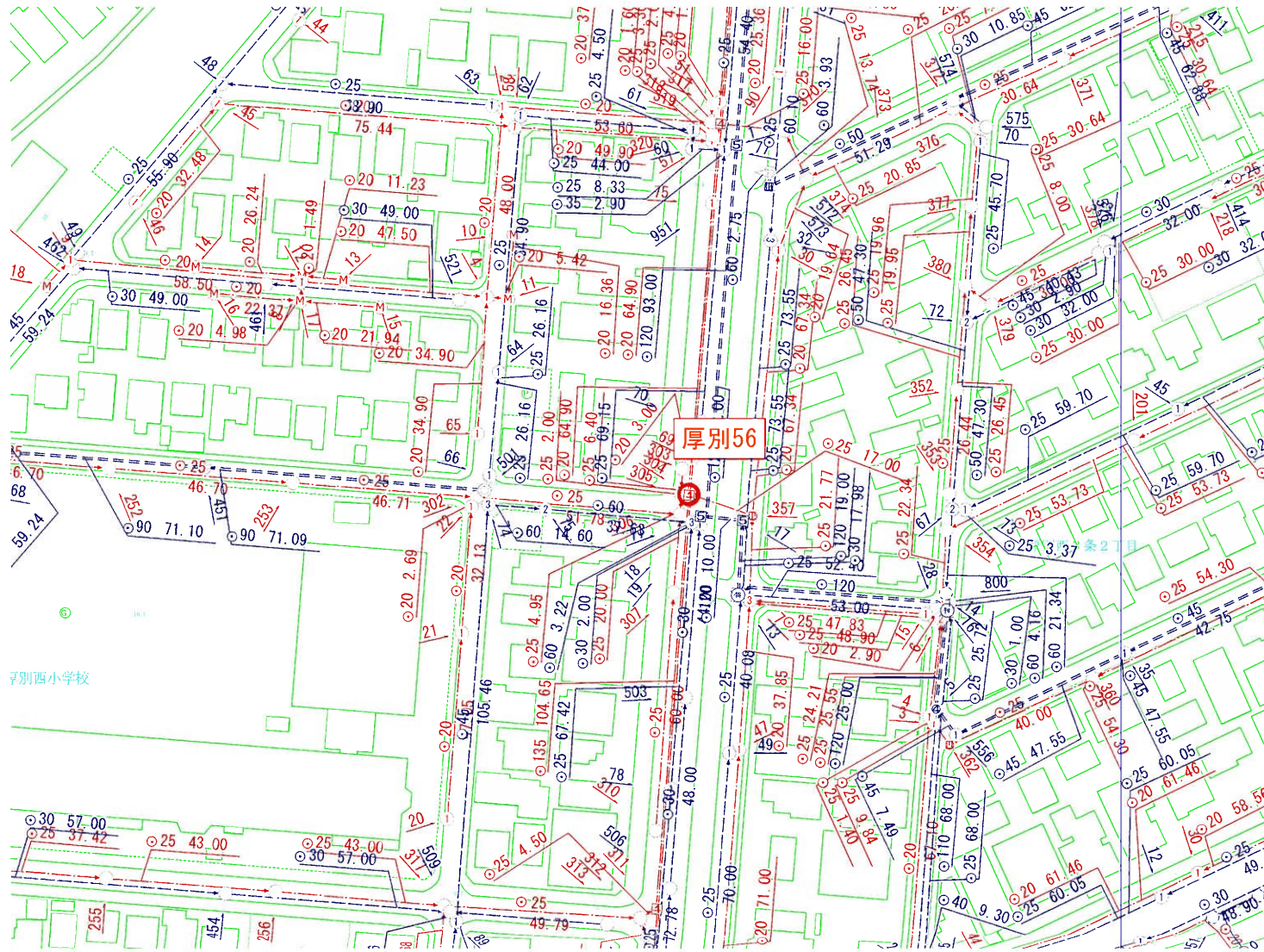
【管路網図】
