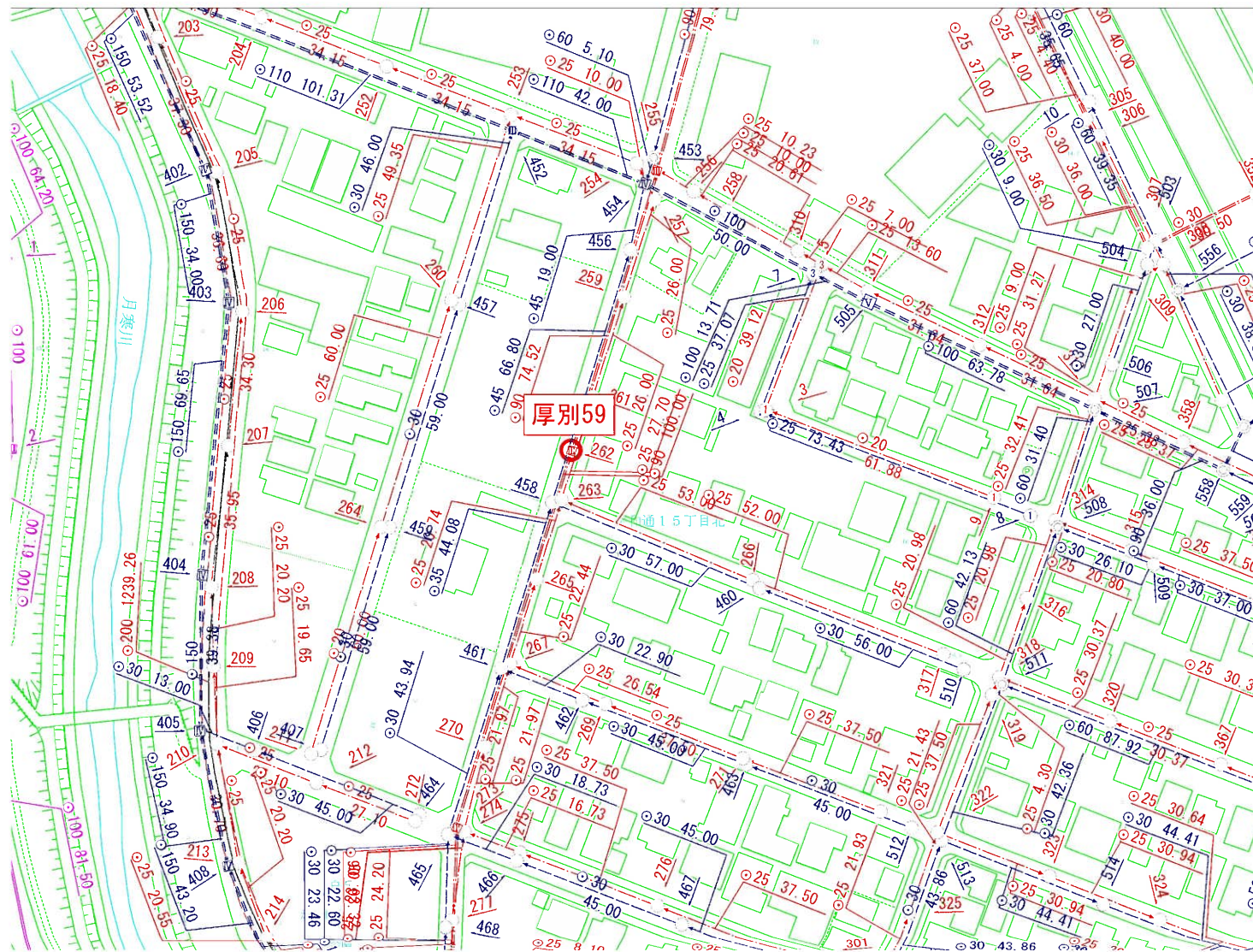
【管路網図】
