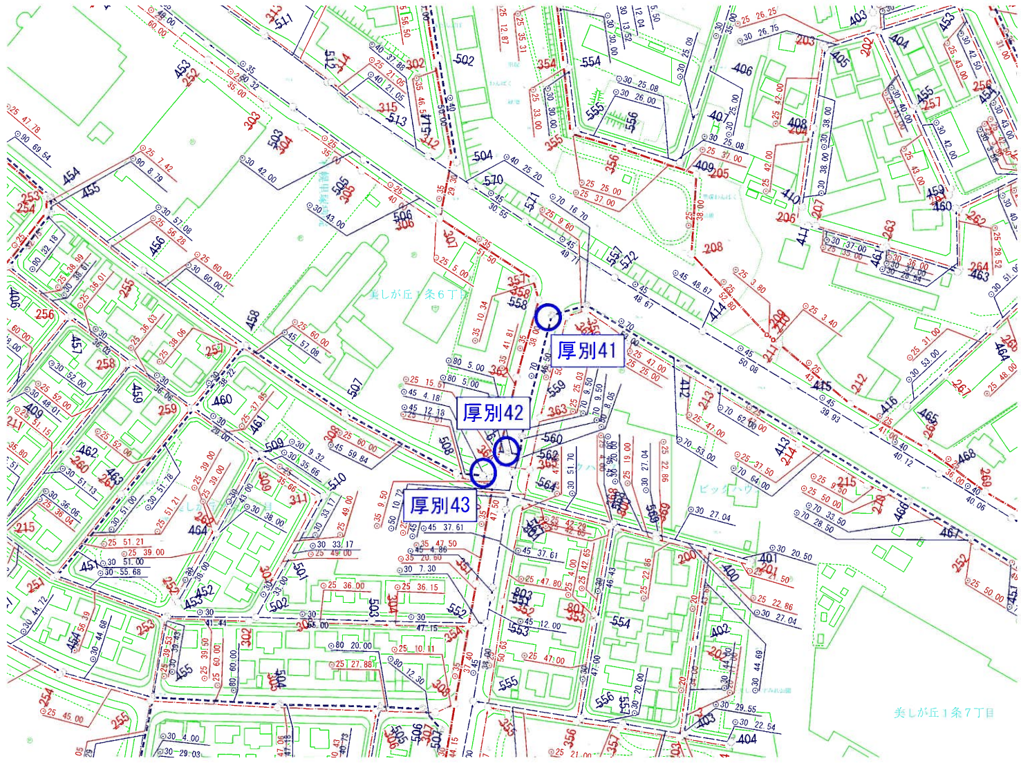
【管路網図】
