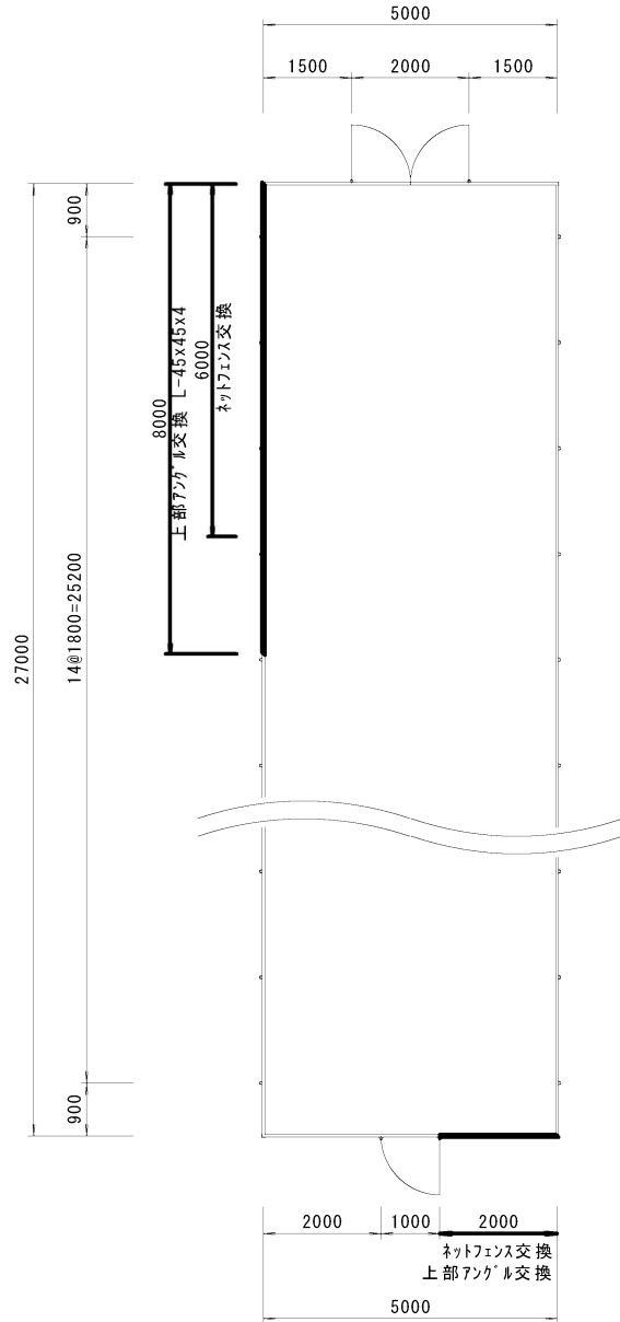
平面図 S=1/100
