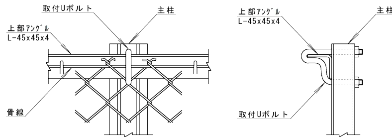
詳細図 S=1/5
