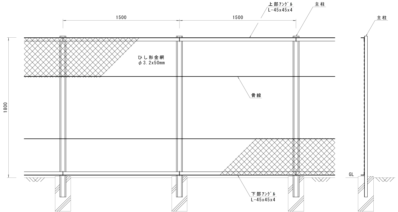
詳細図 S=1/5
