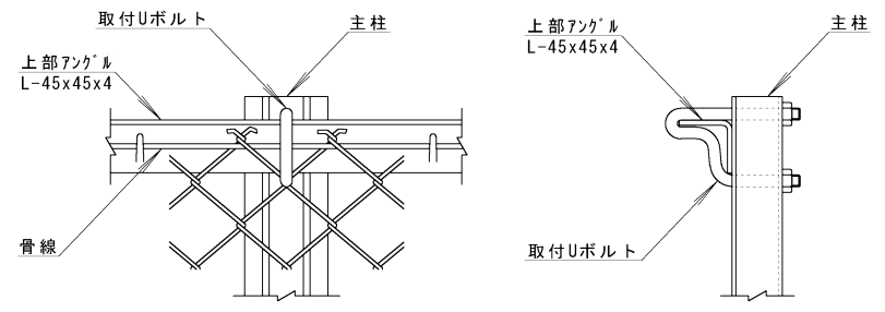
詳細図 S=1/5
