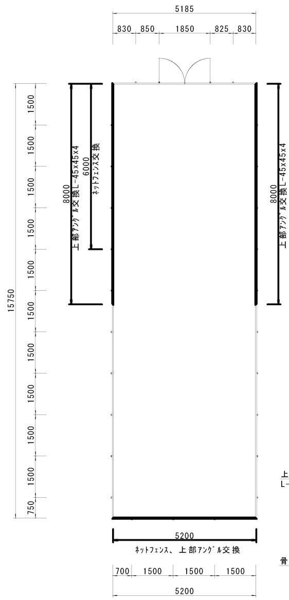
平面図 S=1/100
