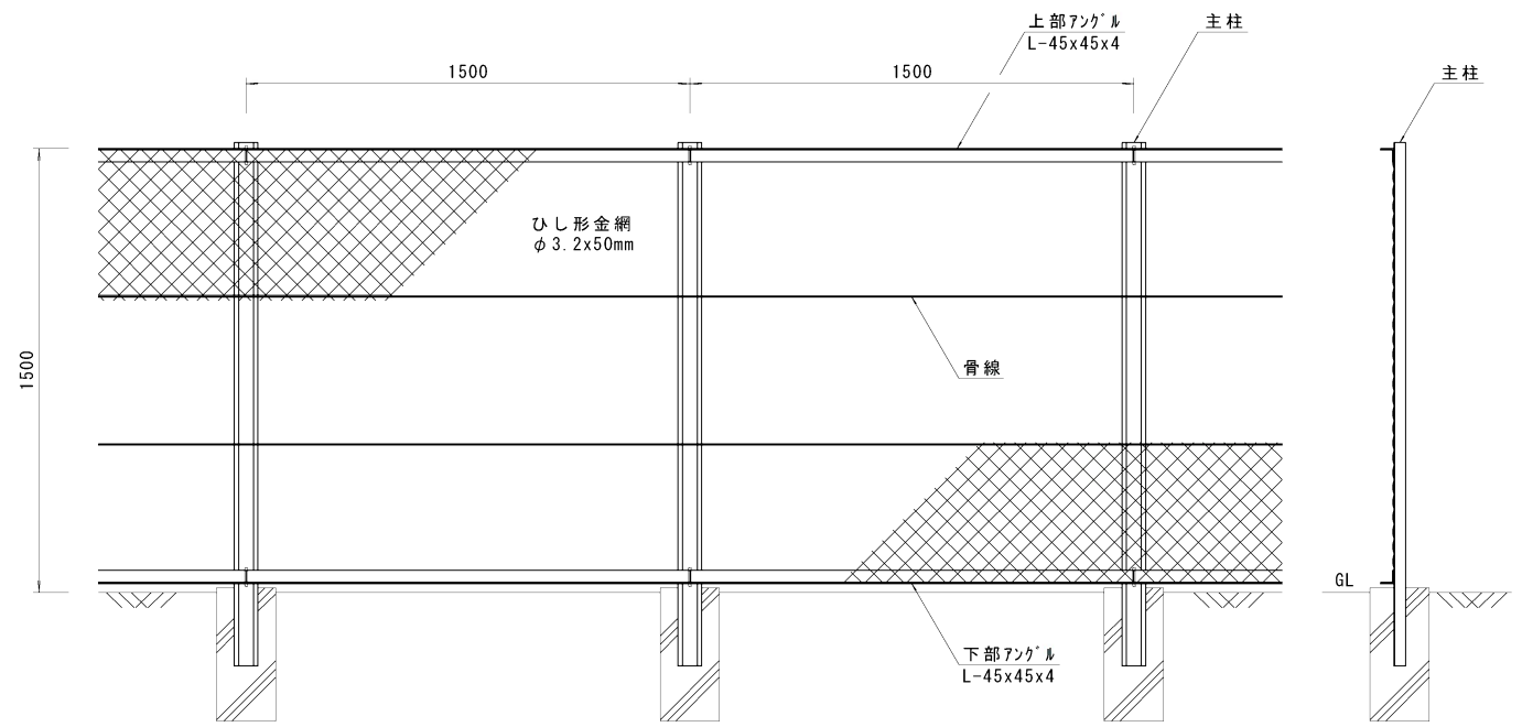
正面図 S=1/20
