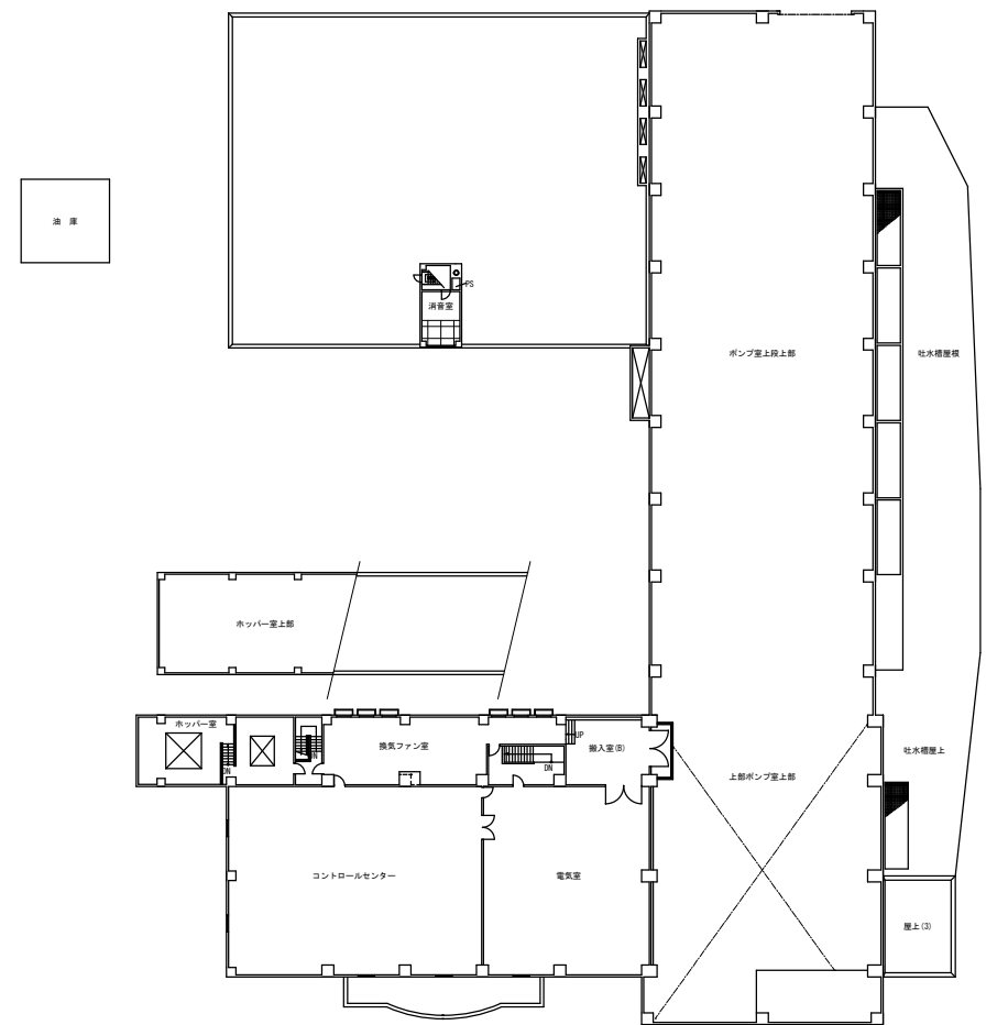
2階平面図
