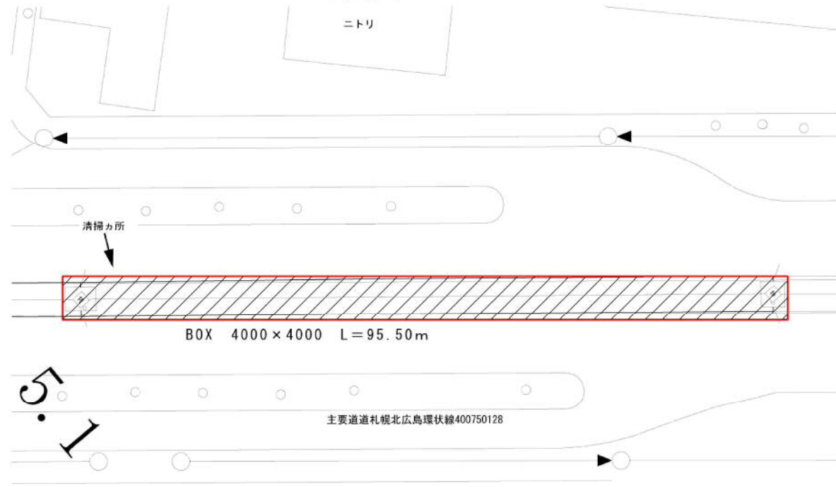
平面図 1 : 500
