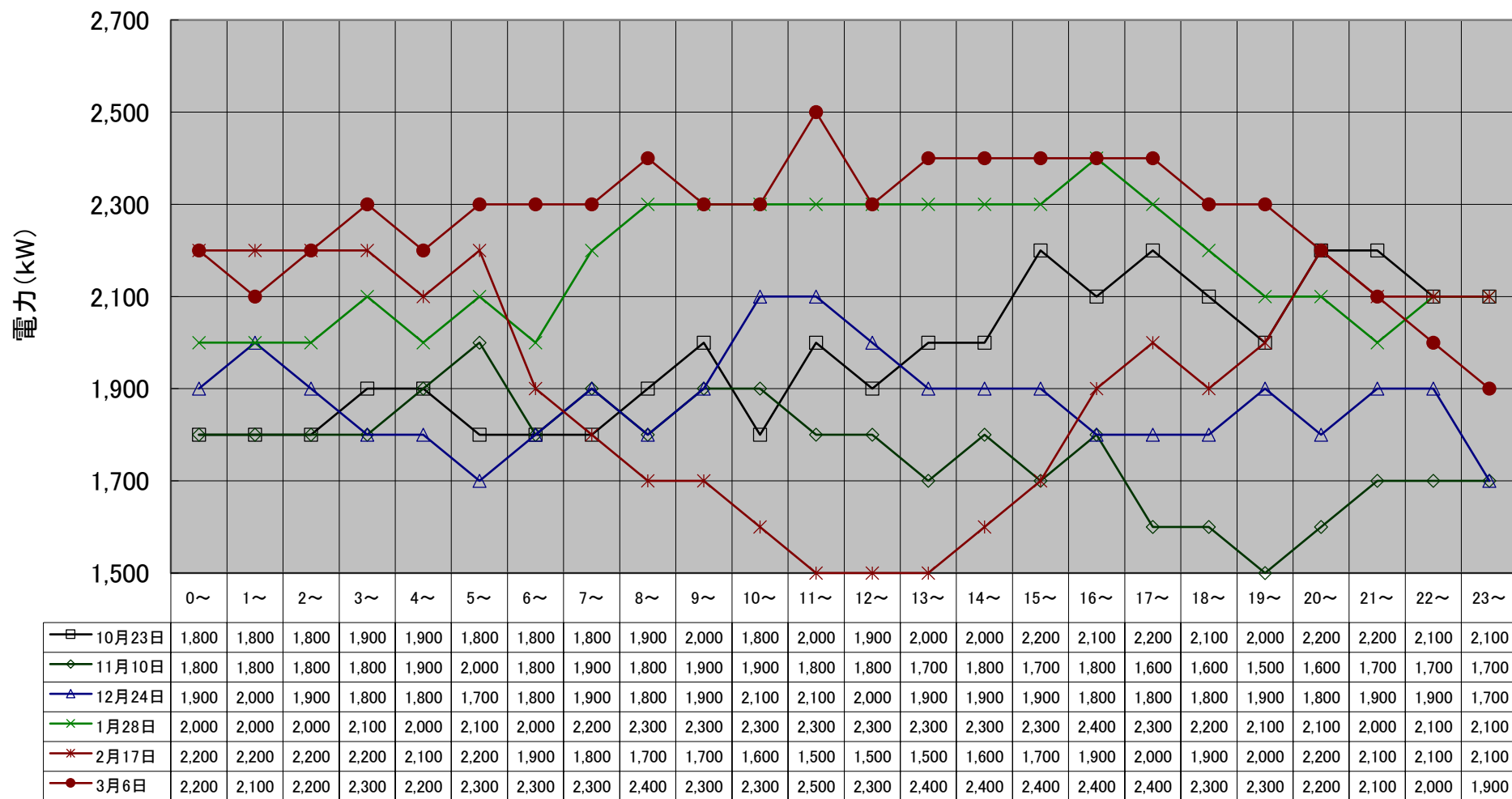
月別最大負荷日ロードカーブ(令和2年度下期)
