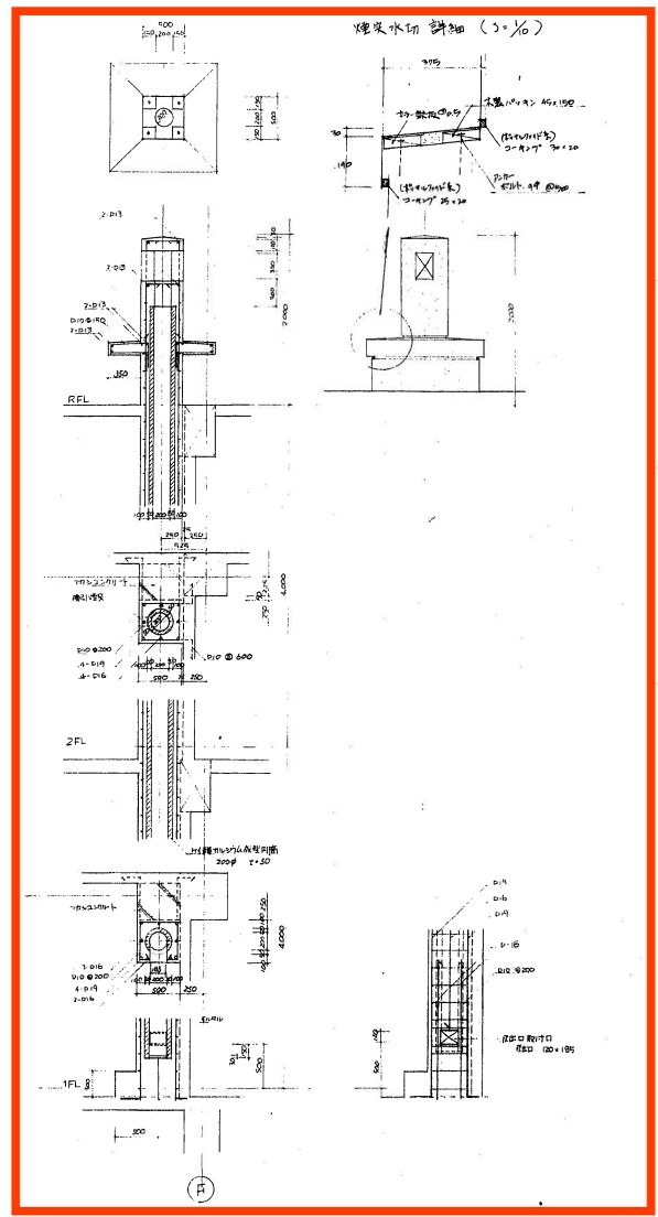
煙灰水研詳圖
