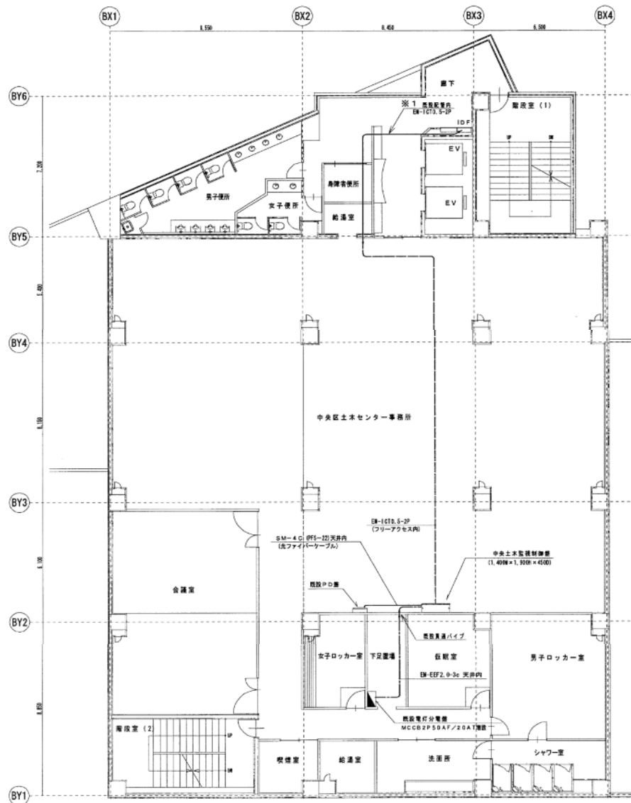
中央区土木部維持管理課配置図
