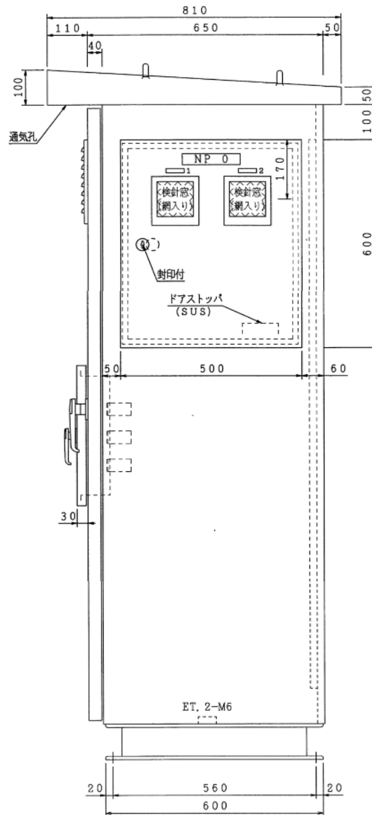
右側面図
