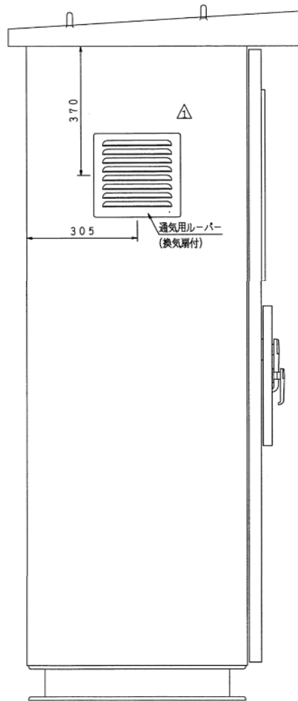
左側面図
