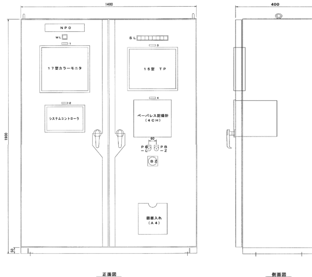
正面図
