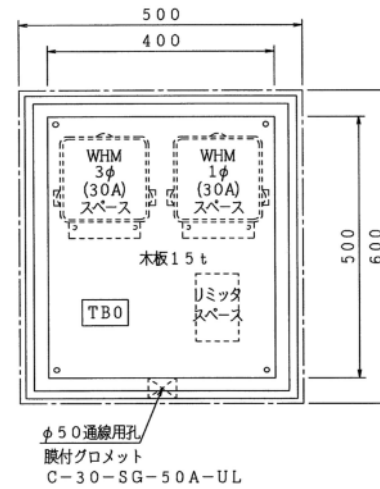
側面内部扉図
