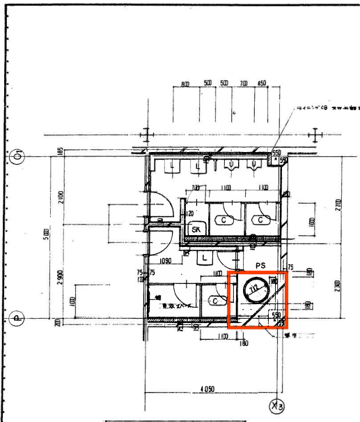
+11.00m 男子トイレ平面詳細図 1:50
