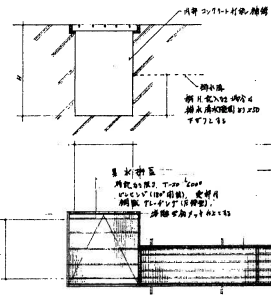
排水設備詳細図 1:20
