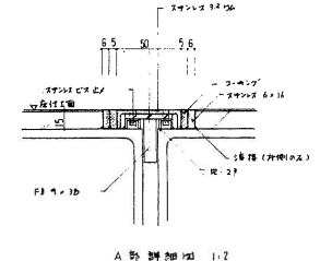
A部詳細図 1:2
