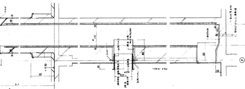
煙突詳細図 1:20
