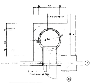
排水設備詳細図 1:20
