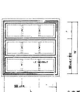
平面図 1:20
