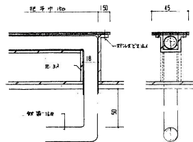
手すり詳細図 1:2
