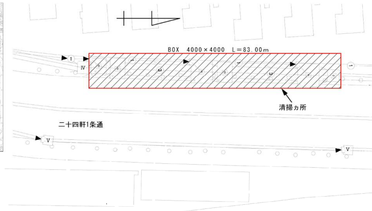
平面図 1 : 500
