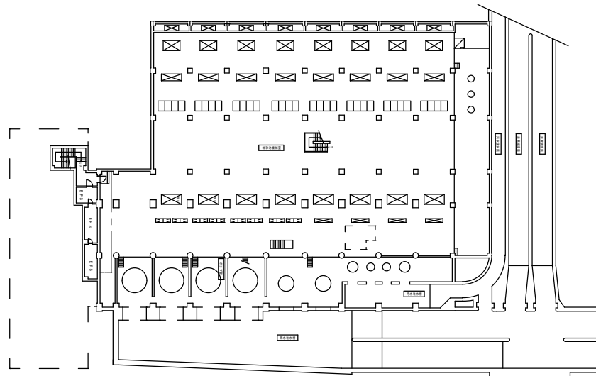
B階全体平面図
