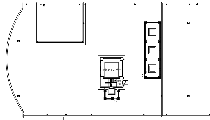
PH階・屋根伏図
