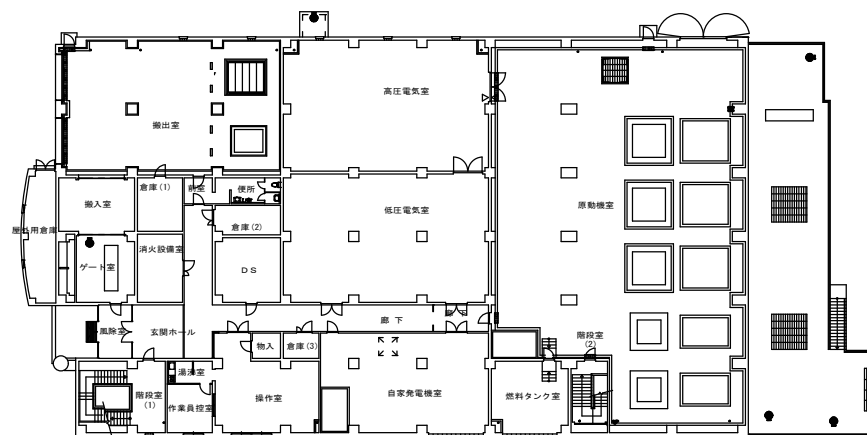
1階 平面図
