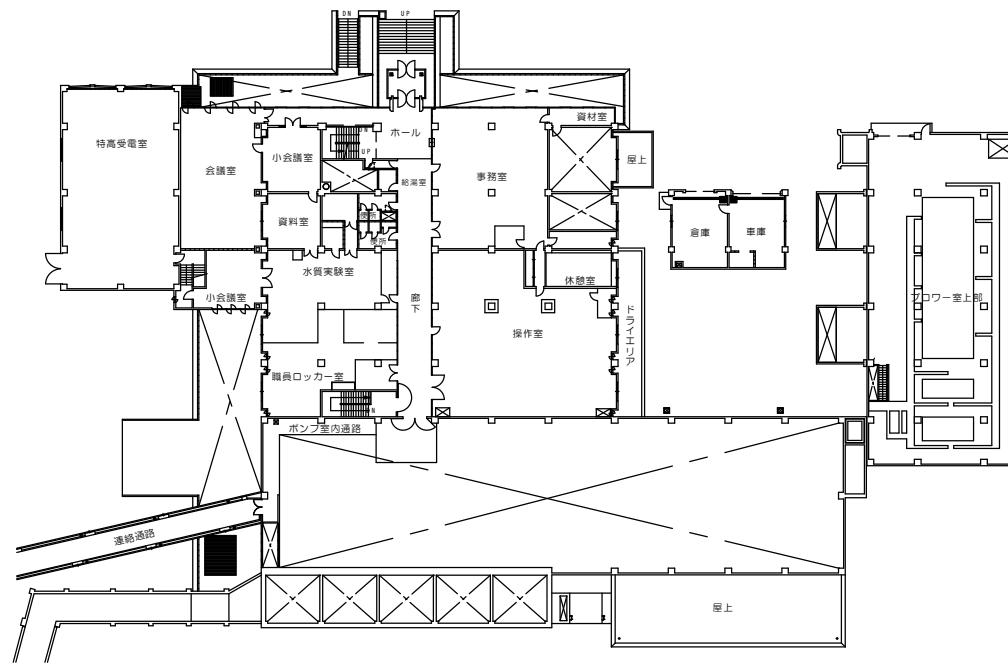
1階
