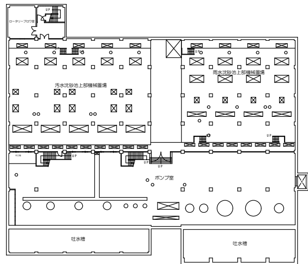
地下2階
