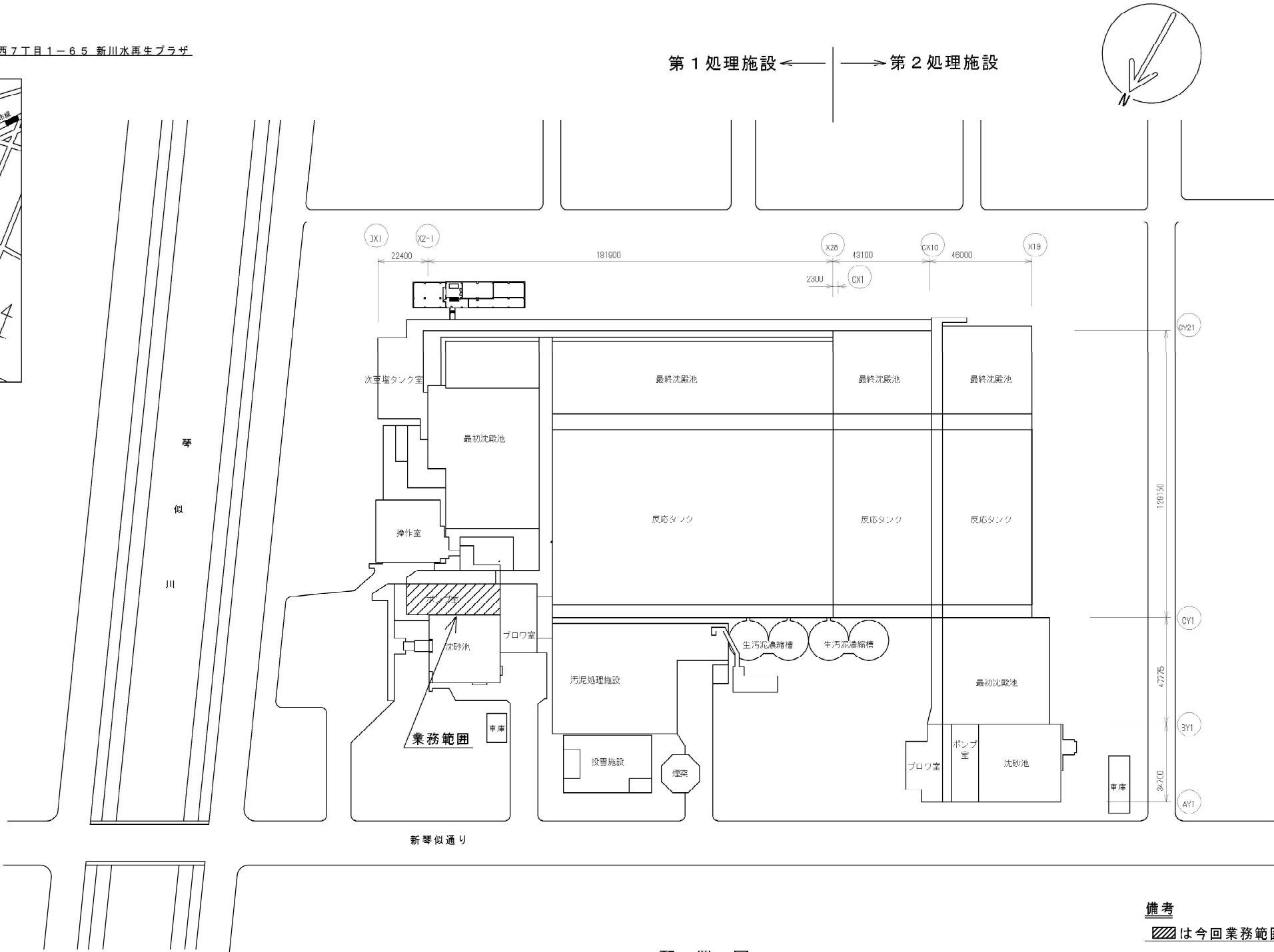
配置図
