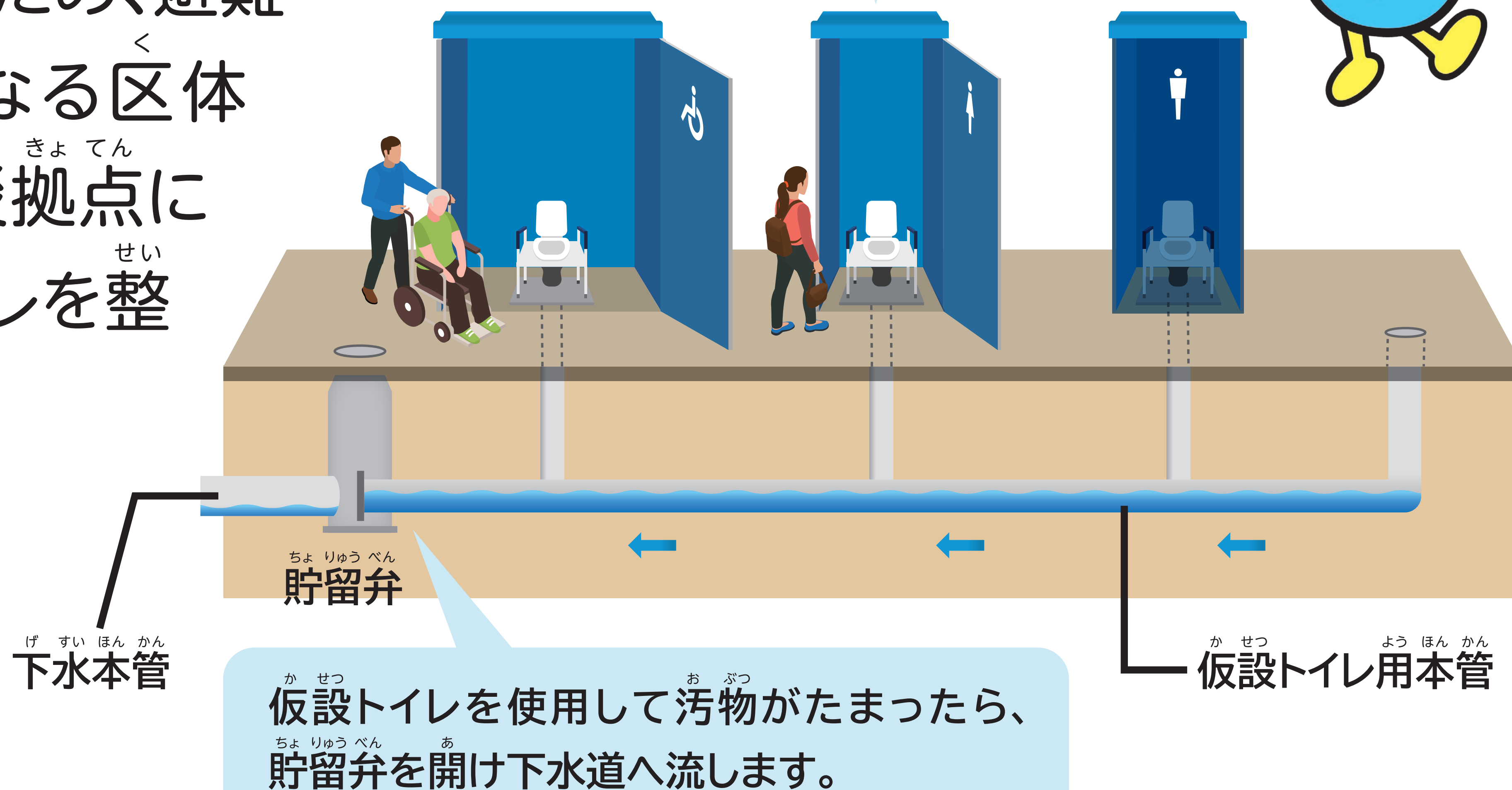
マンホールトイレ
