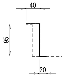
爪金具詳細図
