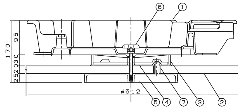
断面図
