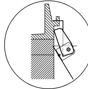
取付詳細図
