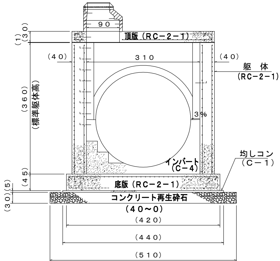
<断面図> S=1/60
