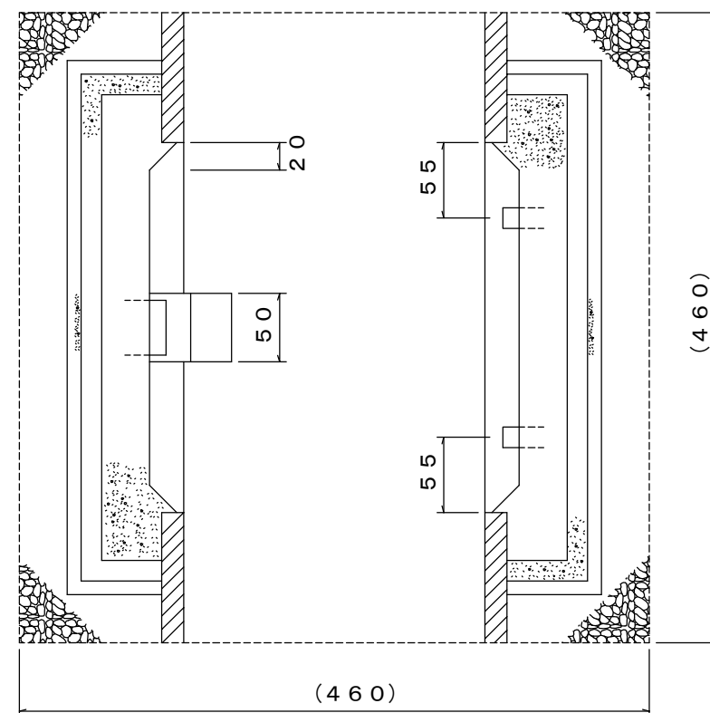
&lt;平面図&gt; S=1/50
