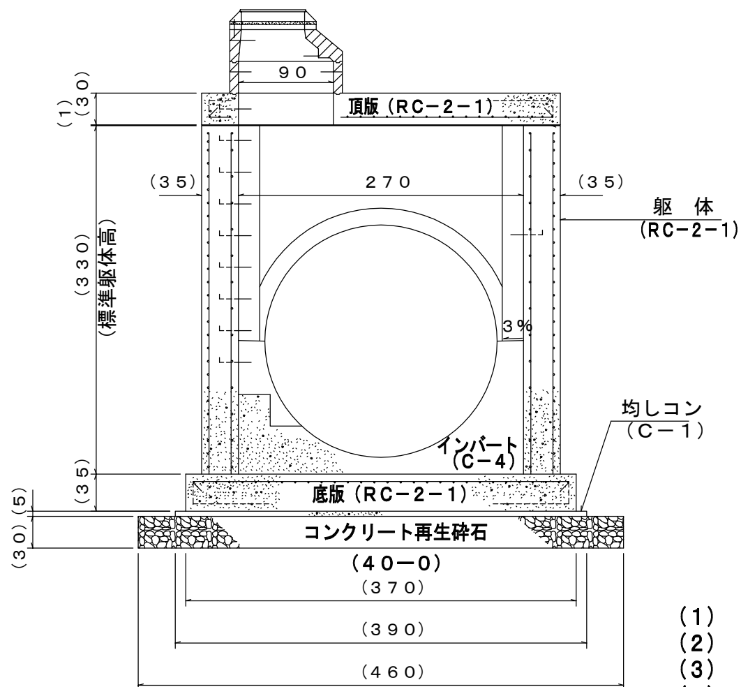
&lt;断面図&gt; S=1/50
