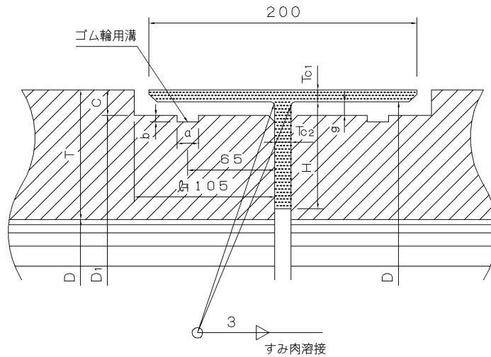
小口径管用カラーの形状
