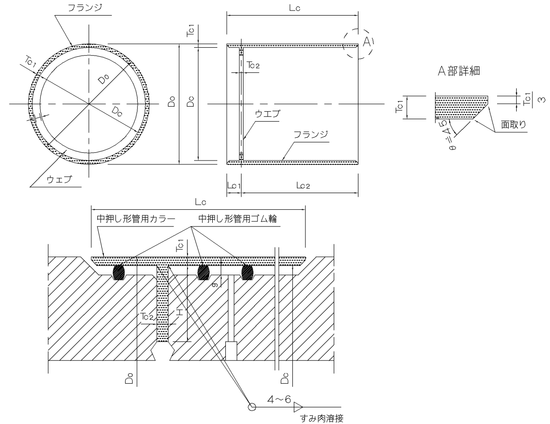
中押し形管用カラーの形状
