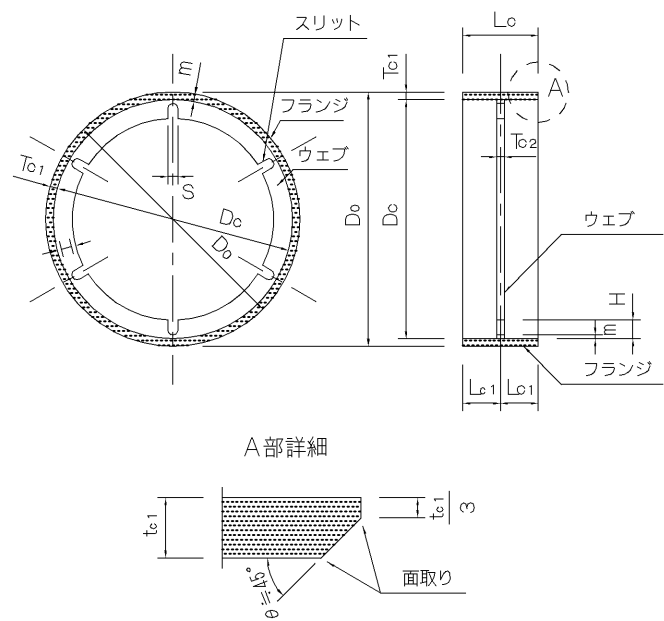
図-1 標準形管用カラーの形状
