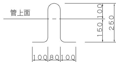
吊りフック詳細
