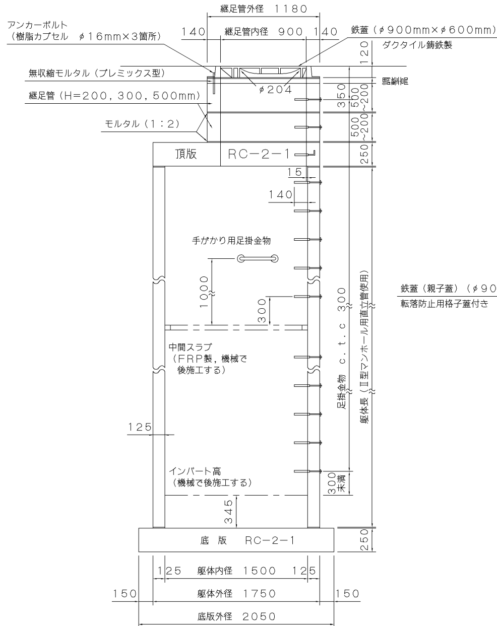
A-A断面図 S=1/40
