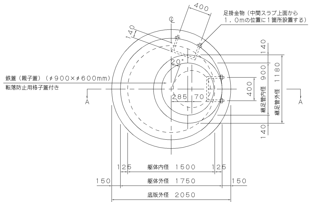
平面図 S=1/40
