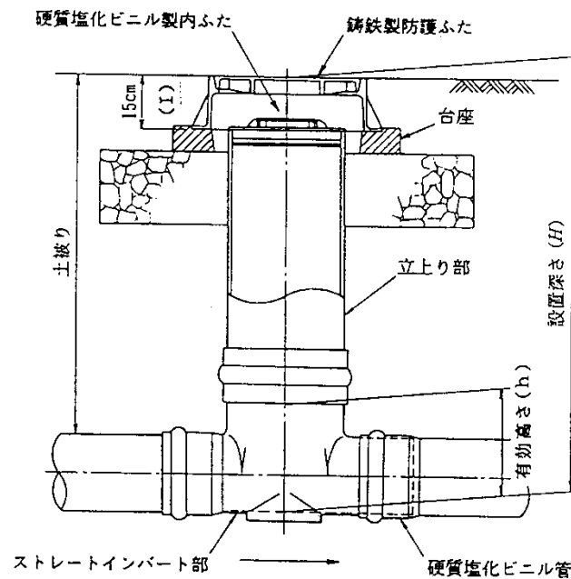
図 - 7 - 4 塩ビ製マシンホール設置図
