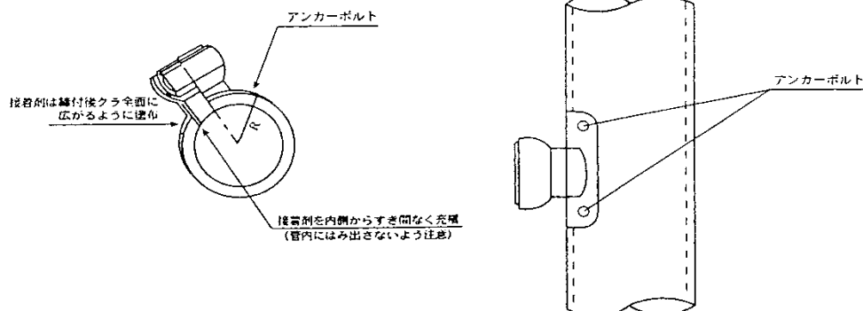
アンカーボルトを使用した場合
