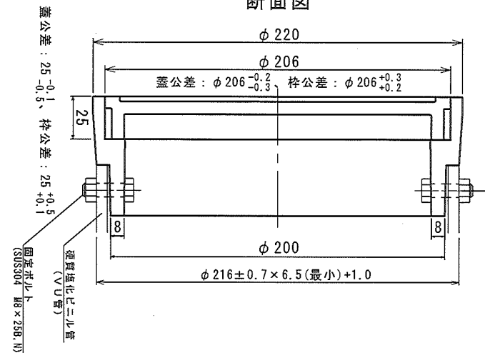
断面図
