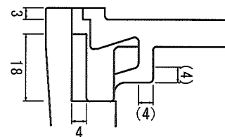
開閉孔拡大図
