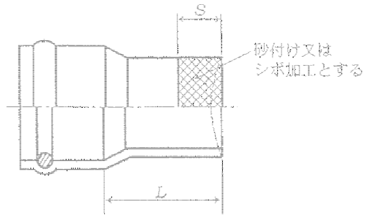
下水道協会規格品 (単位: mm)
