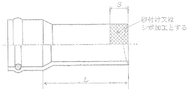
下水道協会規格品 (単位: mm)
